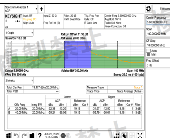
W56 802.11n 20MHz Chain1 5600MHz
