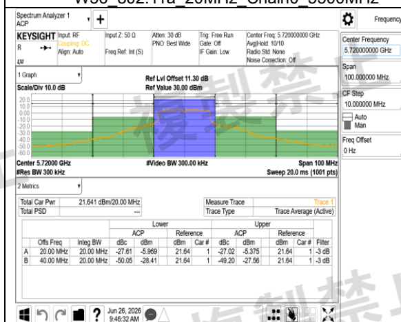
W56 802.11a 20MHz Chain0 5720MHz
