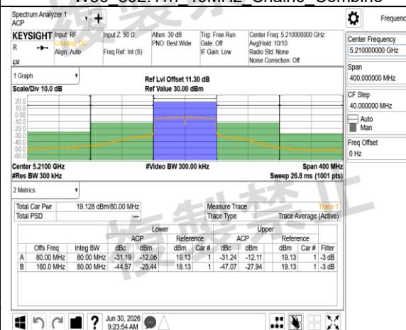
W52 802.11ac 80MHz Chain0 5210MHz
