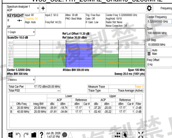
W53 802.11n 20MHz Chain0 5320MHz
