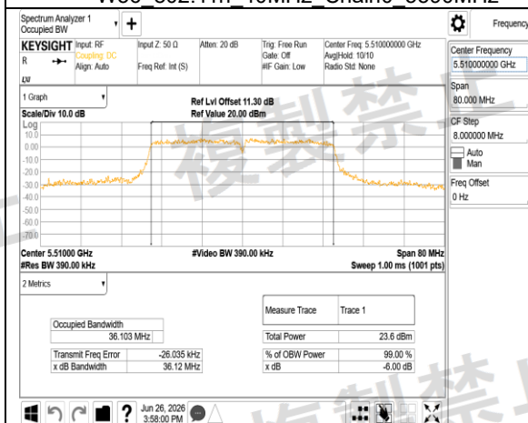
W56 802.11n 40MHz Chain1 5510MHz
