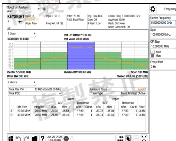
W56 802.11n 20MHz Chain1 5500MHz
