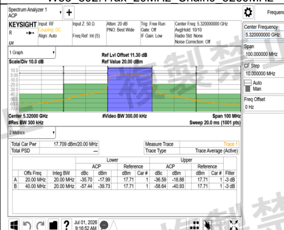
W53 802.11ax 20MHz Chain0 5320MHz
