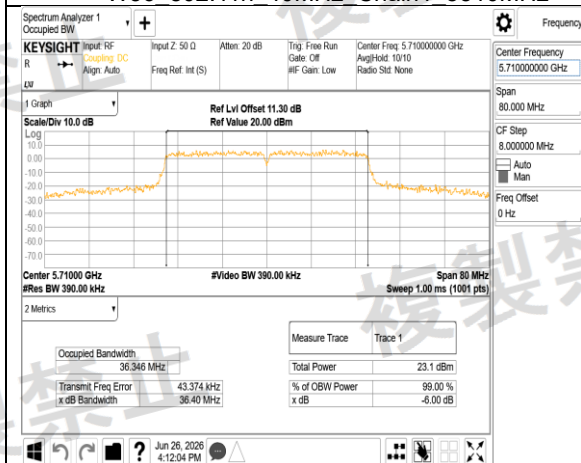
W56 802.11n 40MHz Chain1 5710MHz
