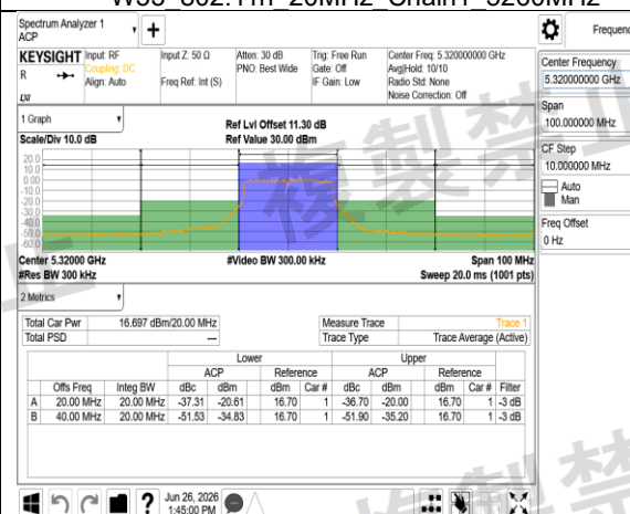
W53 802.11n 20MHz Chain1 5320MHz
