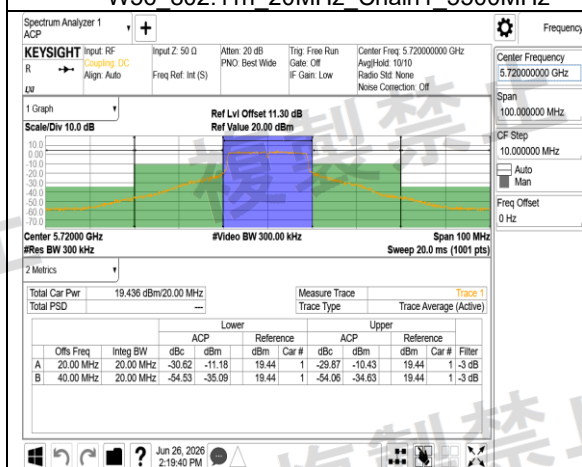
W56 802.11n 20MHz Chain1 5720MHz
