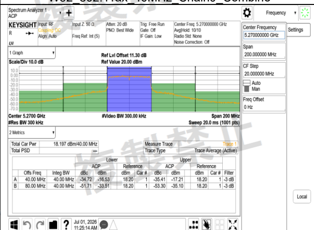
W53 802.11ax 40MHz Chain0 5270MHz
