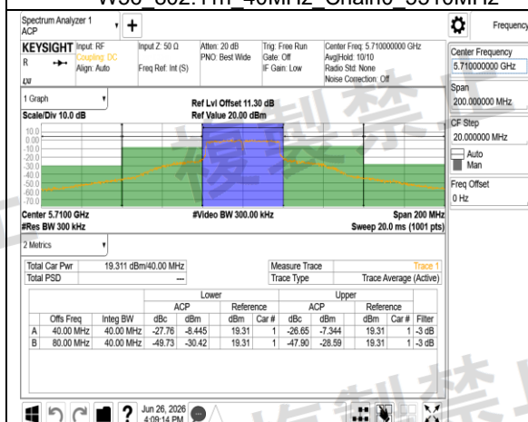
W56 802.11n 40MHz Chain0 5710MHz
