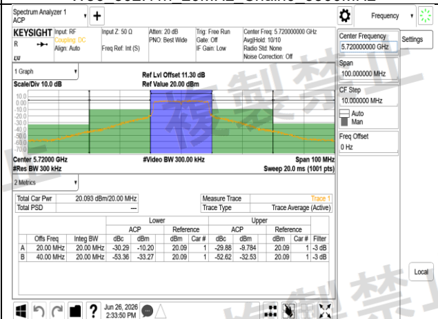
W56 802.11n 20MHz Chain0 5720MHz
