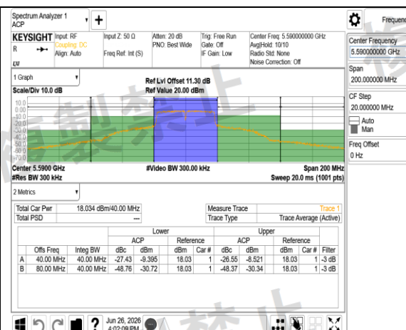
W56 802.11n 40MHz Chain0 5590MHz
