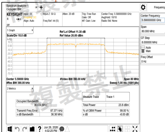
W56 802.11n 40MHz Chain0 5590MHz
