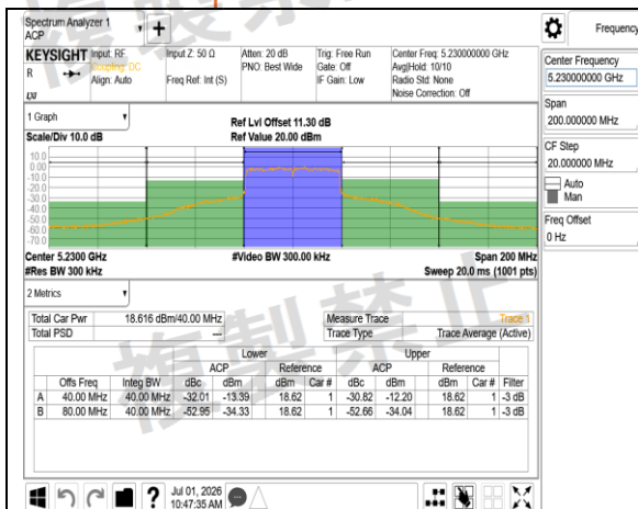
W52 802.11ax 40MHz Chain1 5230MHz
