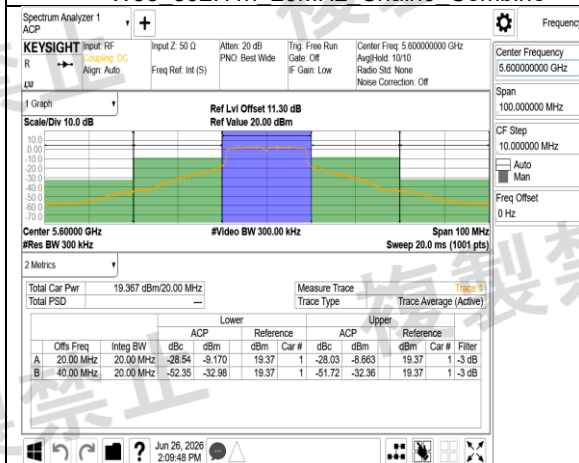
W56 802.11n 20MHz Chain0 5600MHz
