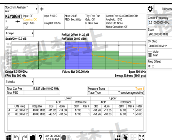
W53 802.11n 40MHz Chain0 5310MHz
