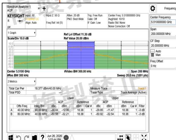
W56 802.11n 40MHz Chain0 5510MHz
