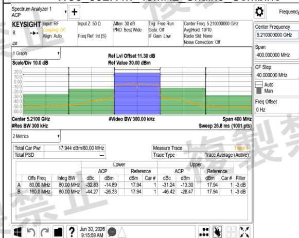
W52 802.11ac 80MHz Chain1 5210MHz
