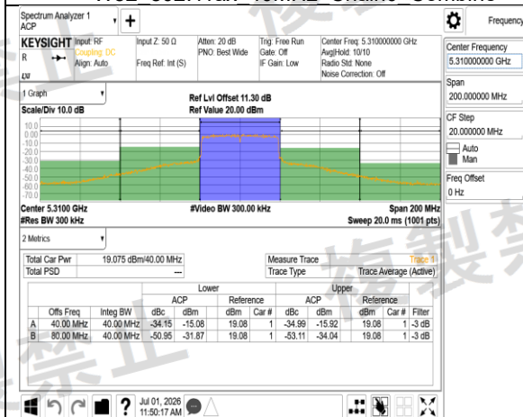
W53 802.11ax 40MHz Chain0 5310MHz
