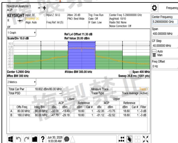
W53 802.11ac 80MHz Chain0 5290MHz
