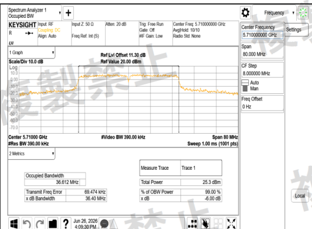
W56 802.11n 40MHz Chain0 5710MHz
