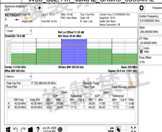
W56 802.11n 40MHz Chain1 5510MHz
