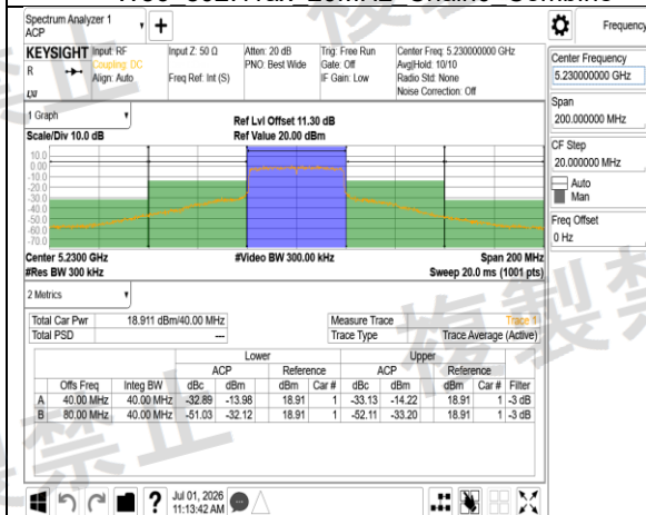
W52 802.11ax 40MHz Chain0 5230MHz
