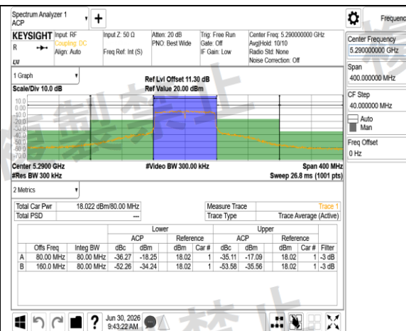
W53 802.11ac 80MHz Chain1 5290MHz
