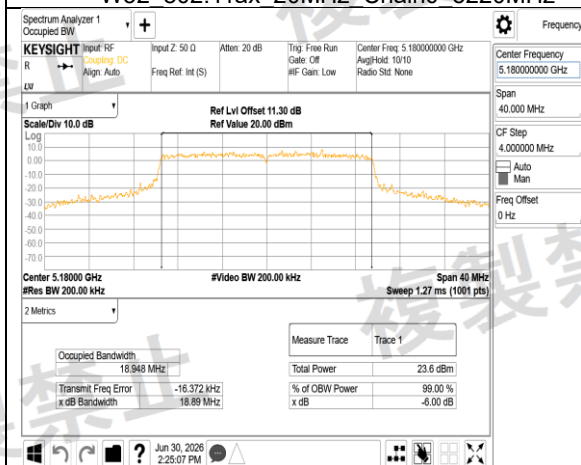
W52 802.11ax 20MHz Chain1 5180MHz
