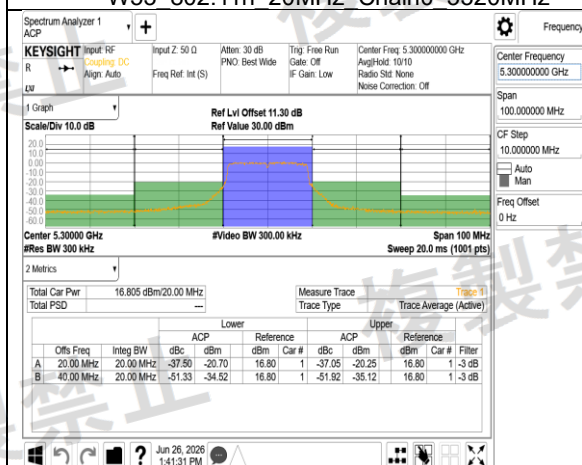
W53 802.11n 20MHz Chain1 5300MHz
