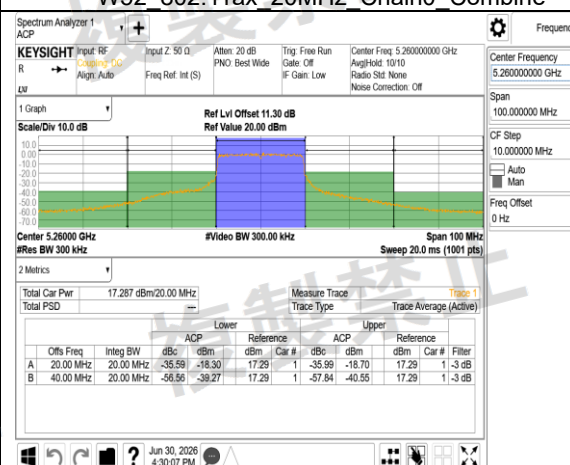
W53 802.11ax 20MHz Chain0 5260MHz
