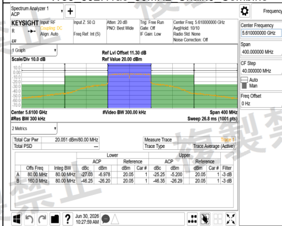
W56 802.11ac 80MHz Chain0 5610MHz
