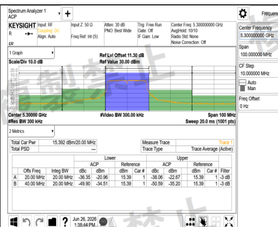
W53 802.11n 20MHz Chain0 5300MHz
