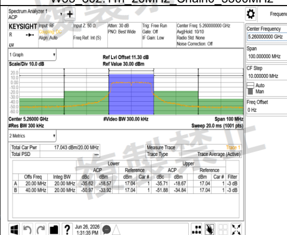
W53 802.11n 20MHz Chain1 5260MHz
