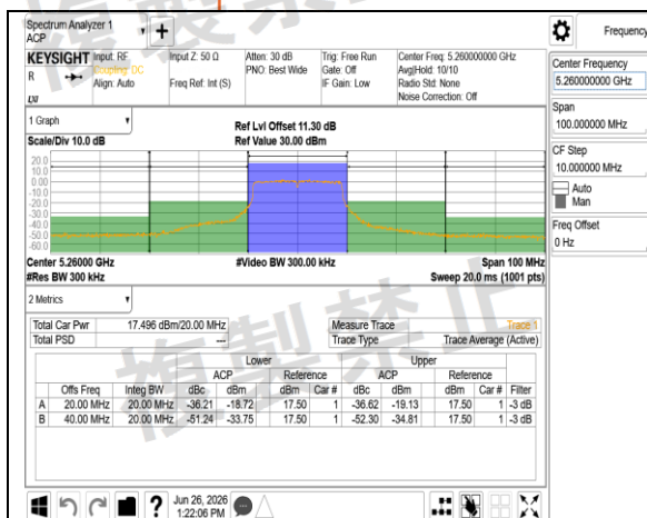
W53 802.11n 20MHz Chain0 5260MHz
