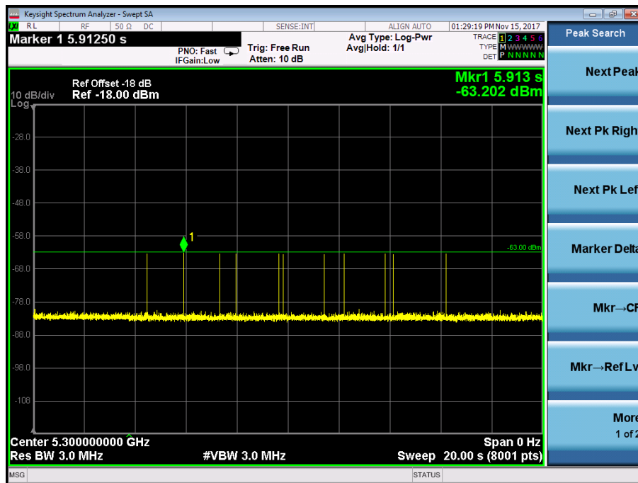
雷達測試信號 Type #6 校驗圖 for 5300MHz
