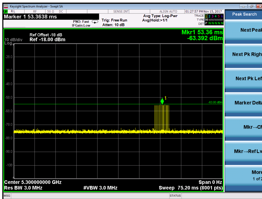
雷達測試信號 Type #4 校驗圖 for 5300MHz
