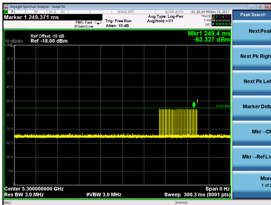
雷達測試信號 Type #1(Test A)校驗圖 for 5300MHz
