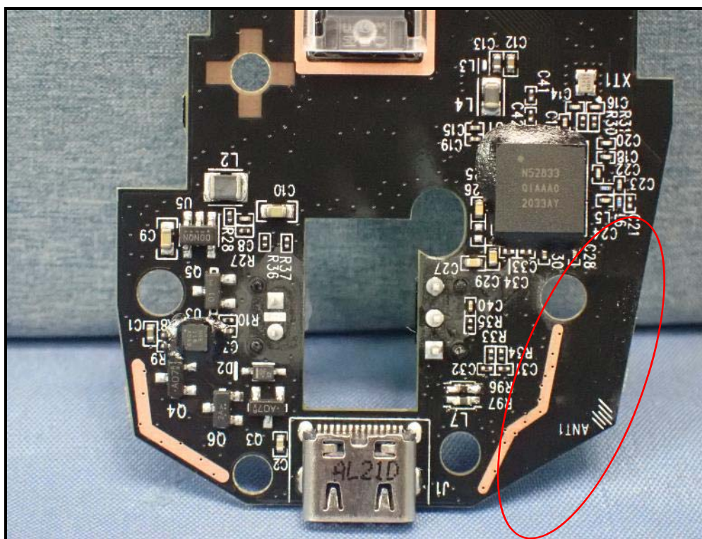
Antenna
