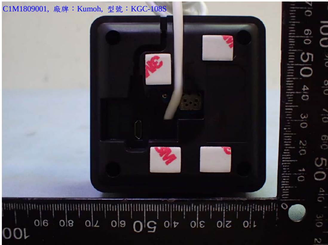
照片 6 外觀 (底部)
