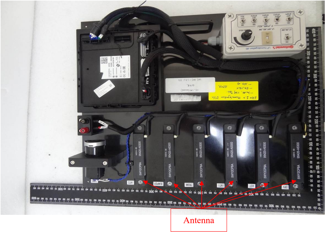
EUT 2
