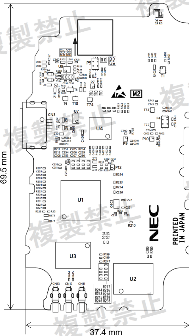
【半田面】
