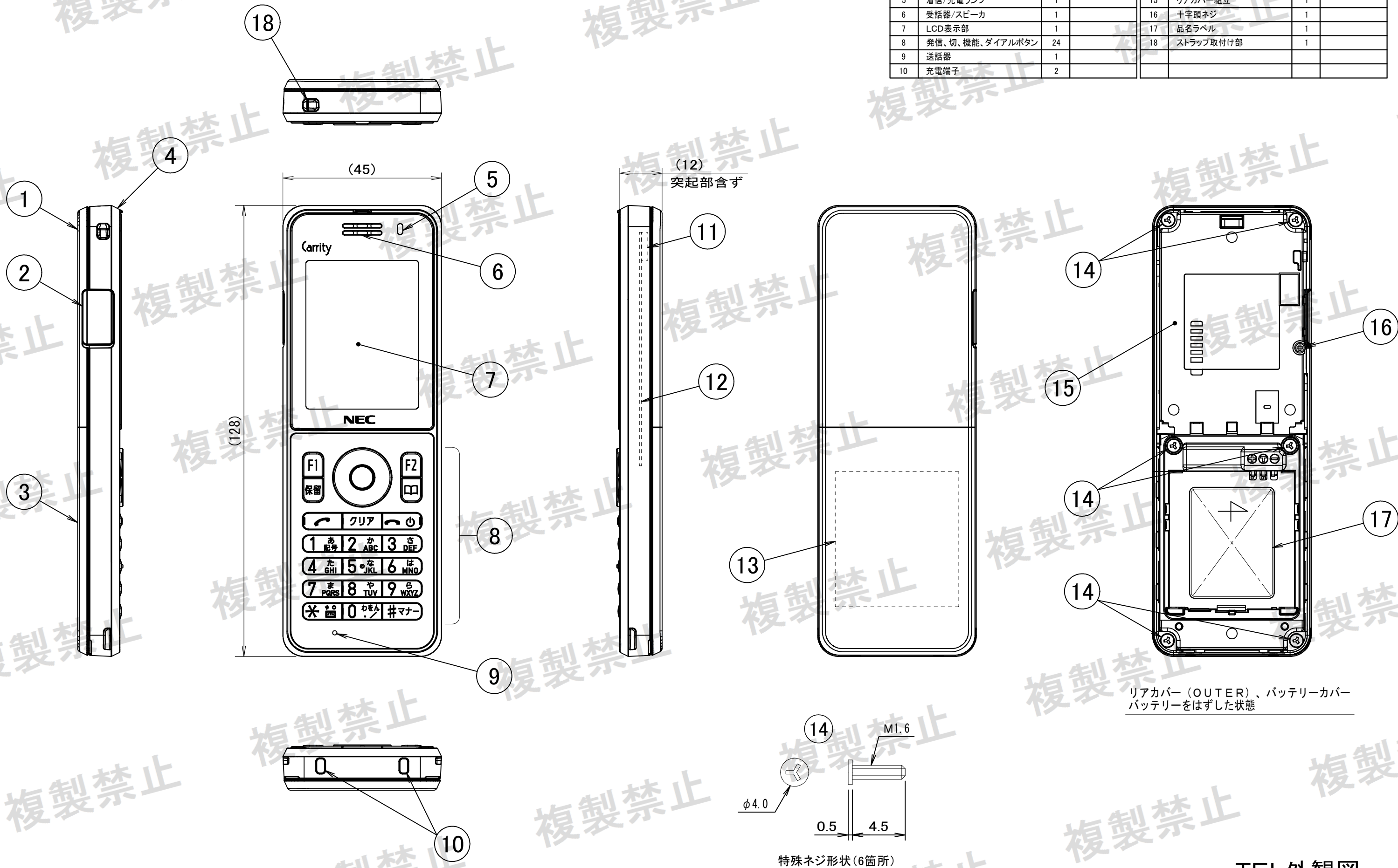
TEL外観図
