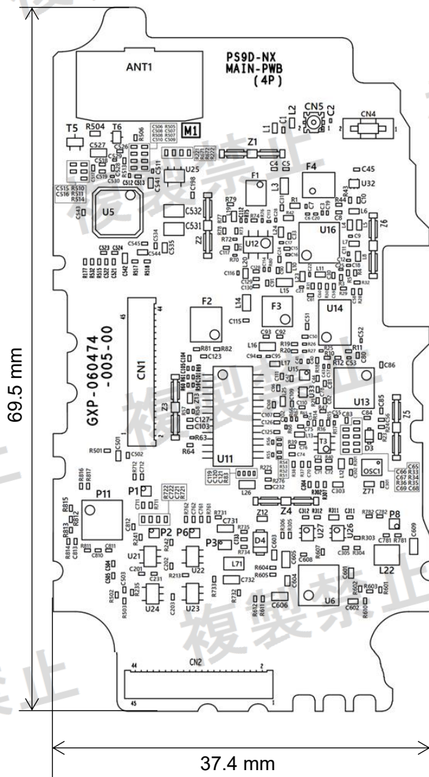
【部品面】
