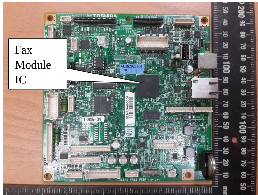
相片二：FAX Module 銅軌面
