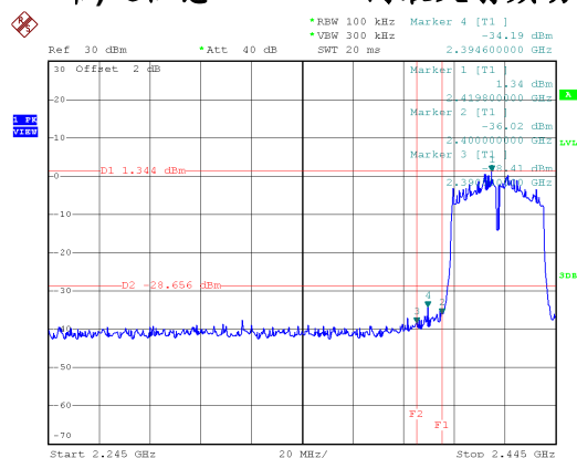
IEEE 802.11n (HT40)頻帶範圍外(下邊緣頻帶)之任意 100 kHz 內最大射頻功率
