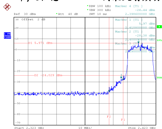
IEEE 802.11n (HT20)頻帶範圍外(下邊緣頻帶)之任意 100 kHz 內最大射頻功率
