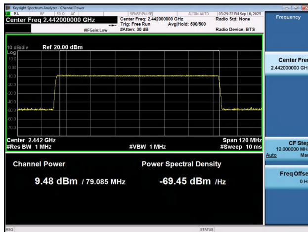
NTNV-2DH5-Ant1-Hop-PASS
