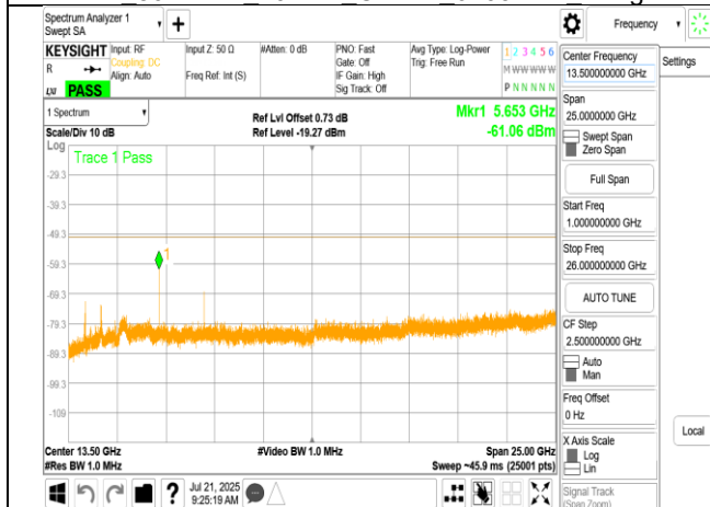
LPI 802.11be 40MHz Chain1 6405MHz Range2
