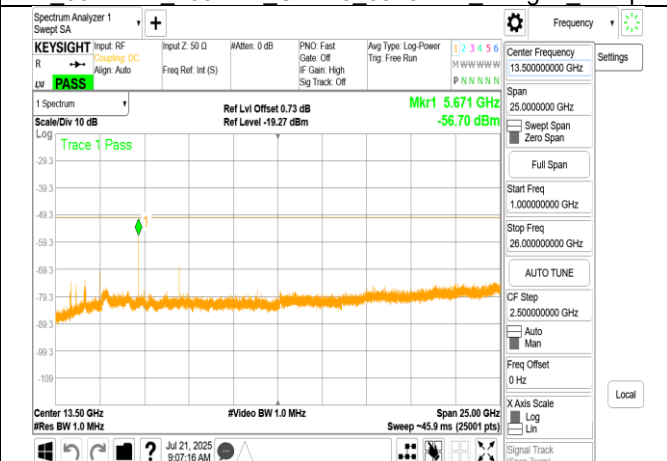
LPI 802.11ax 160MHz Chain1 6025MHz Range2
