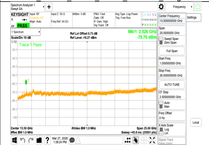
VLP 802.11a 20MHz Chain0 6175MHz Range2
