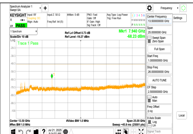
LPI 802.11be 20MHz Chain1 5955MHz Range2
