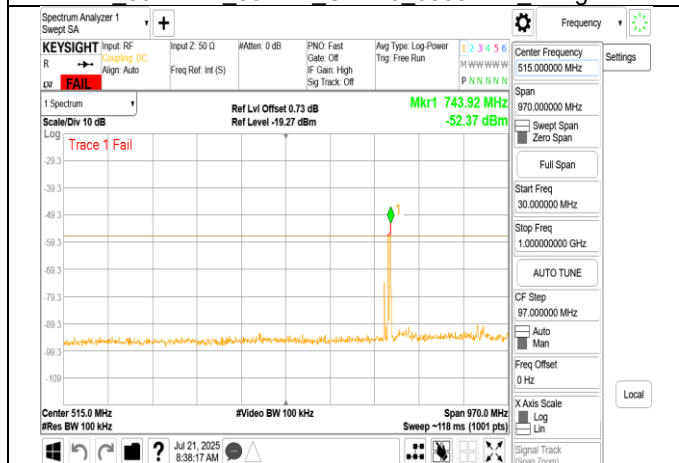
LPI 802.11ac 80MHz Chain1 5985MHz Range1
