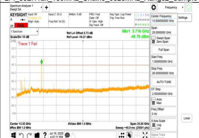
LPI 802.11ax 160MHz Chain0 6185MHz Range2
