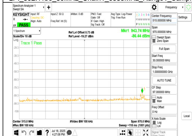
LPI 802.11be 160MHz Chain0 6025MHz Range1
