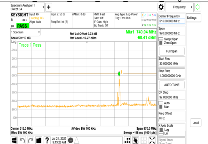
LPI 802.11be 20MHz Chain1 5955MHz Range1
