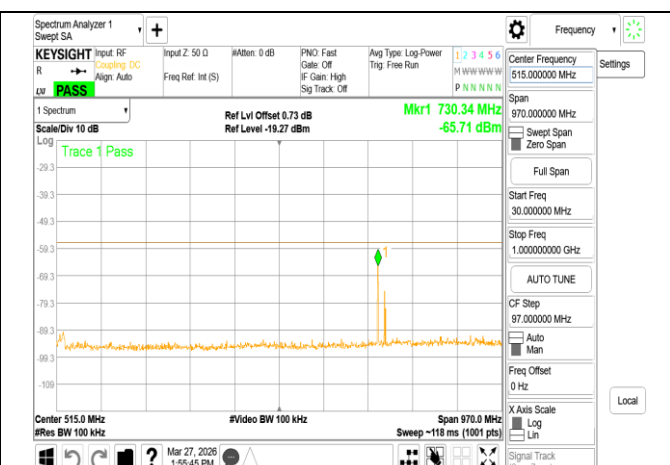
VLP 802.11n 40MHz Chain0 5965MHz Range1
