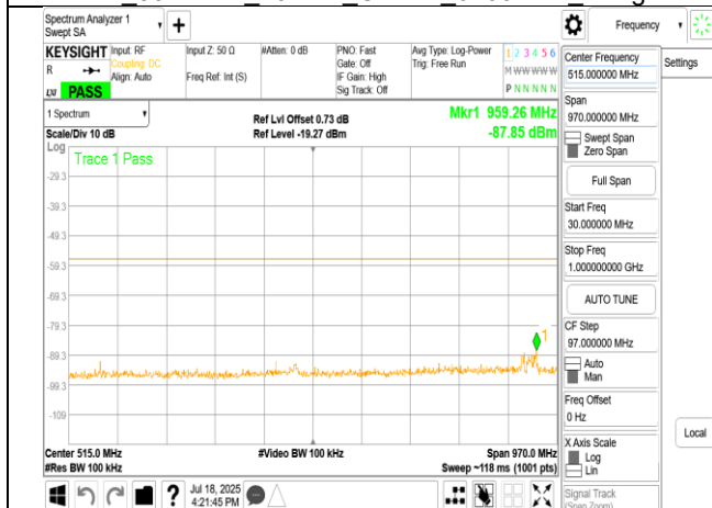
LPI 802.11be 80MHz Chain0 5985MHz Range1
