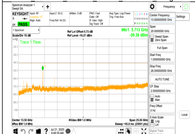
LPI 802.11ac 160MHz Chain1 6345MHz Range2
