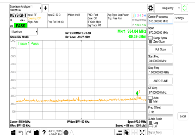
LPI 802.11ax 160MHz Chain0 6025MHz Range1
