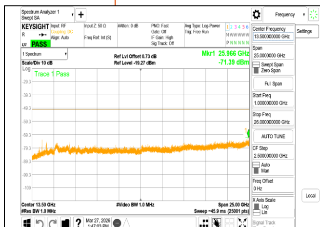
VLP 802.11n 20MHz Chain1 5955MHz Range2
