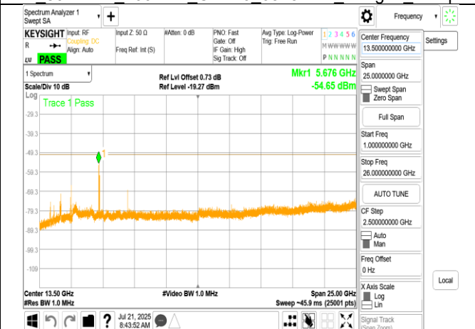
LPI 802.11ac 160MHz Chain1 6025MHz Range2
