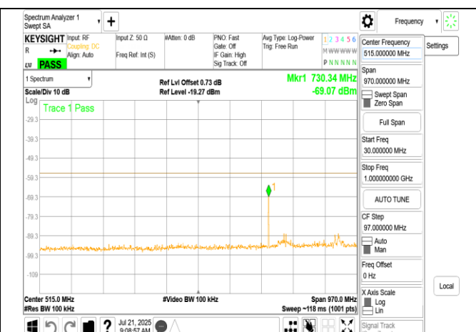
LPI 802.11ax 160MHz Chain1 6185MHz Range1
