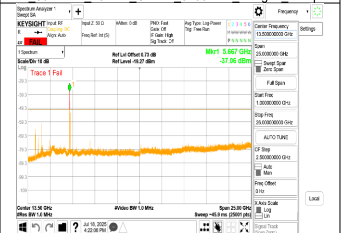
LPI 802.11be 80MHz Chain0 5985MHz Range2
