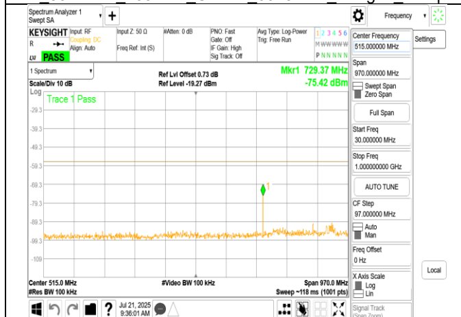
LPI 802.11be 160MHz Chain1 6185MHz Range1
