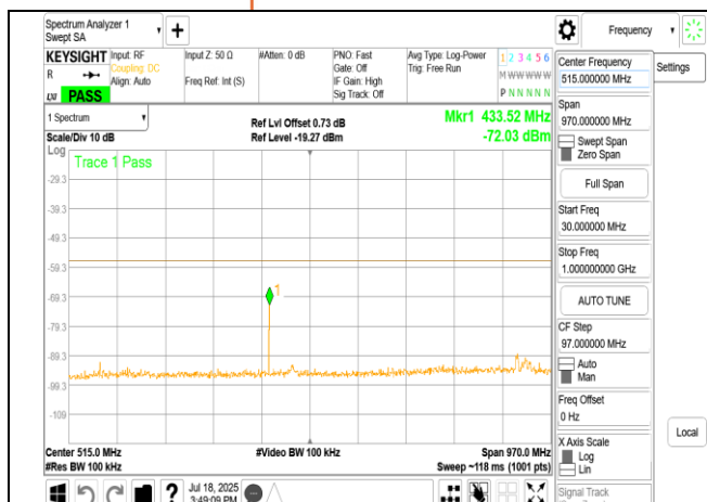
LPI 802.11ax 20MHz Chain0 5955MHz Range1
