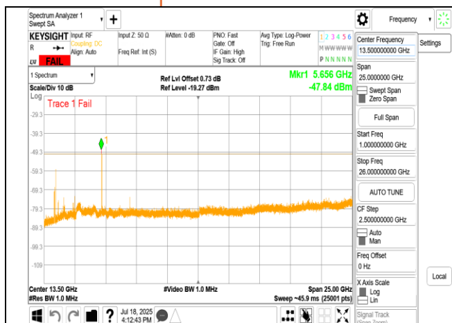
LPI 802.11be 20MHz Chain0 6175MHz Range2
