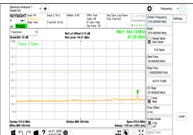
LPI 802.11ac 80MHz Chain1 6145MHz Range1
