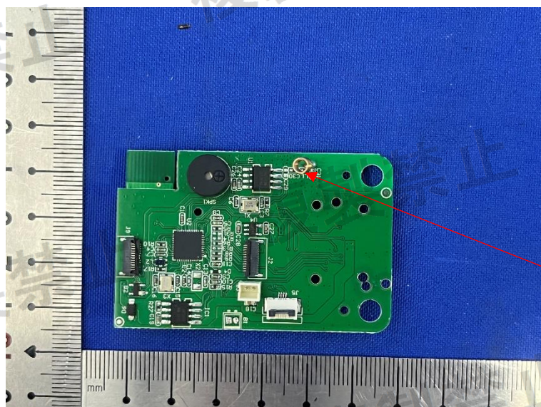
2.4G ANT
