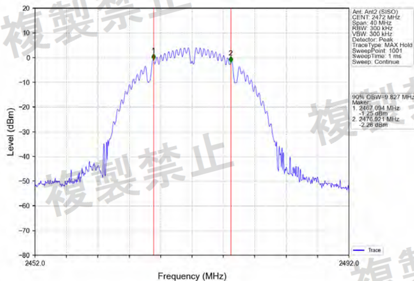
802.11b_2472MHz_Ant2 (SISO)_NTNV
