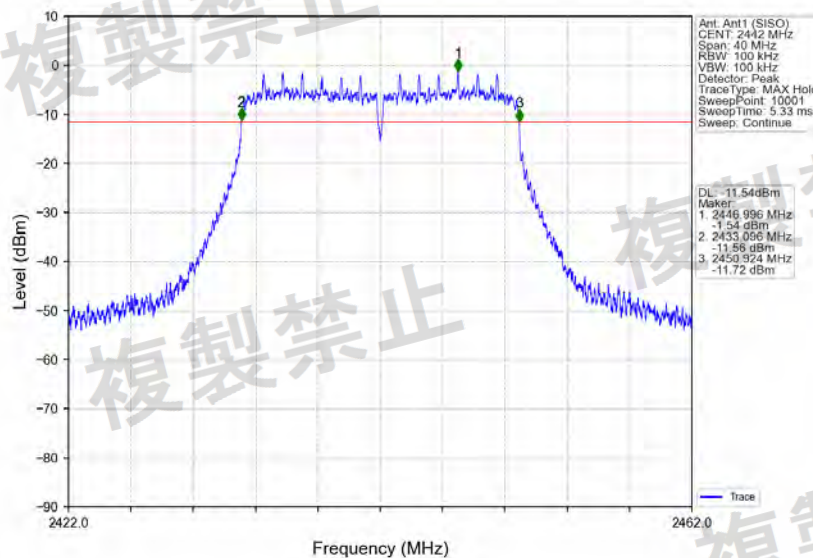
802.11n(HT20)_2442MHz_Ant1 (SISO)_NTNV
