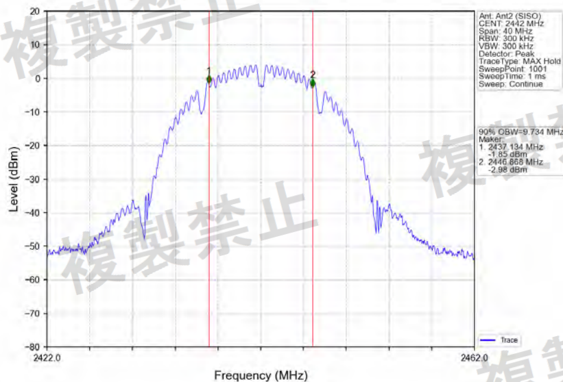
802.11b_2442MHz_Ant2 (SISO)_NTNV
