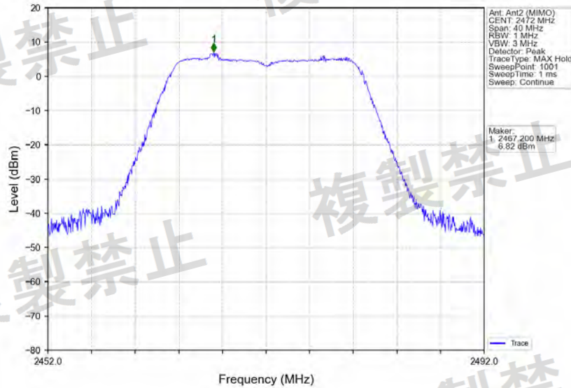
802.11n(HT20)_2472MHz_Ant2 (MIMO)_NTNV
