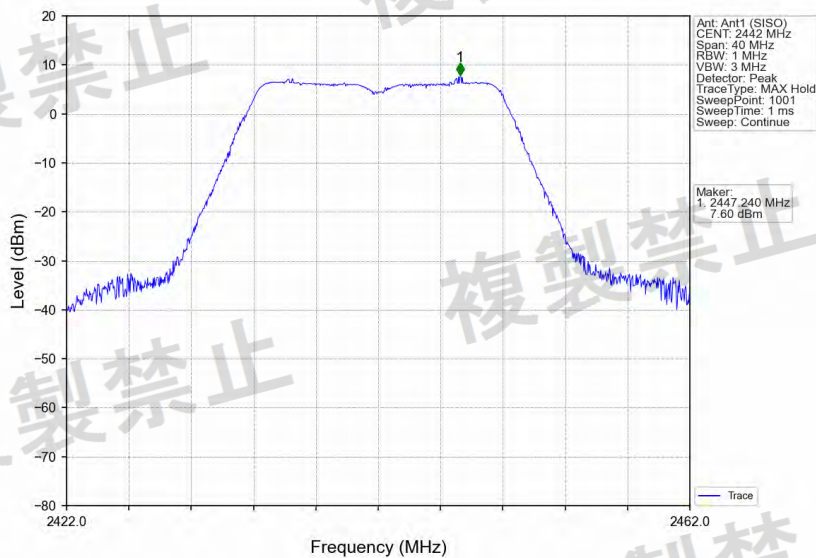
802.11g_2442MHz_Ant1 (SISO)_NTNV
