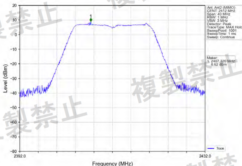
802.11n(HT20)_2412MHz_Ant2 (MIMO)_NTNV
