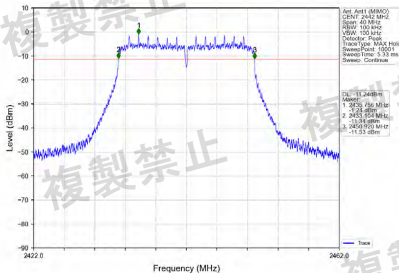
802.11n(HT20)_2442MHz_Ant1 (MIMO)_NTNV
