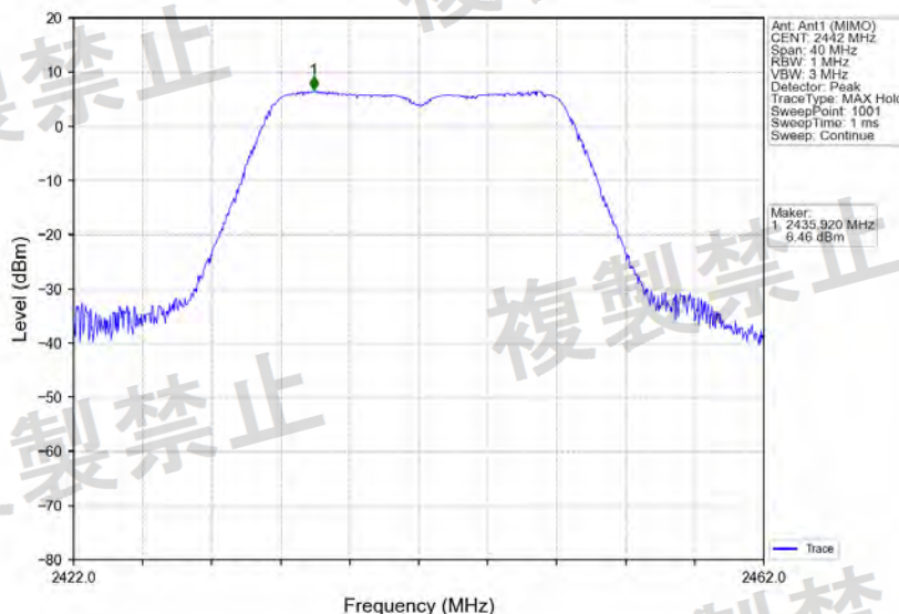
802.11n(HT20)_2442MHz_Ant1 (MIMO)_NTNV
