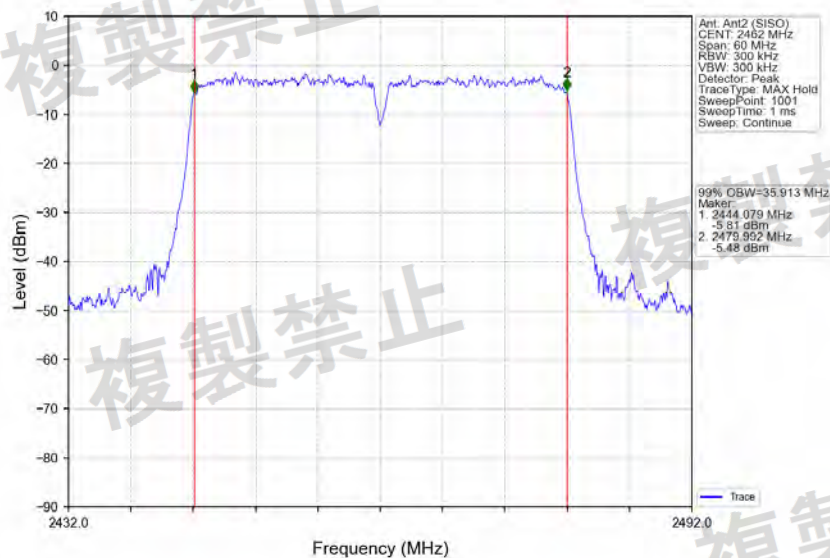
802.11n(HT40)_2462MHz_Ant2 (SISO)_NTNV
