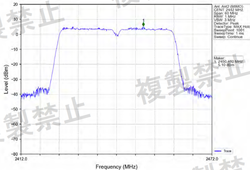
802.11n(HT40)_2442MHz_Ant2 (MIMO)_NTNV
