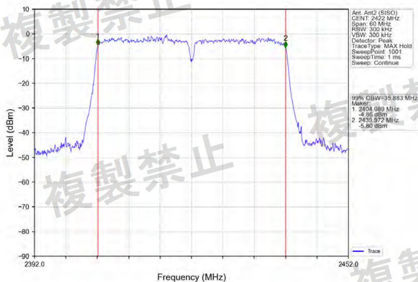
802.11n(HT40)_2422MHz_Ant2 (SISO)_NTNV
