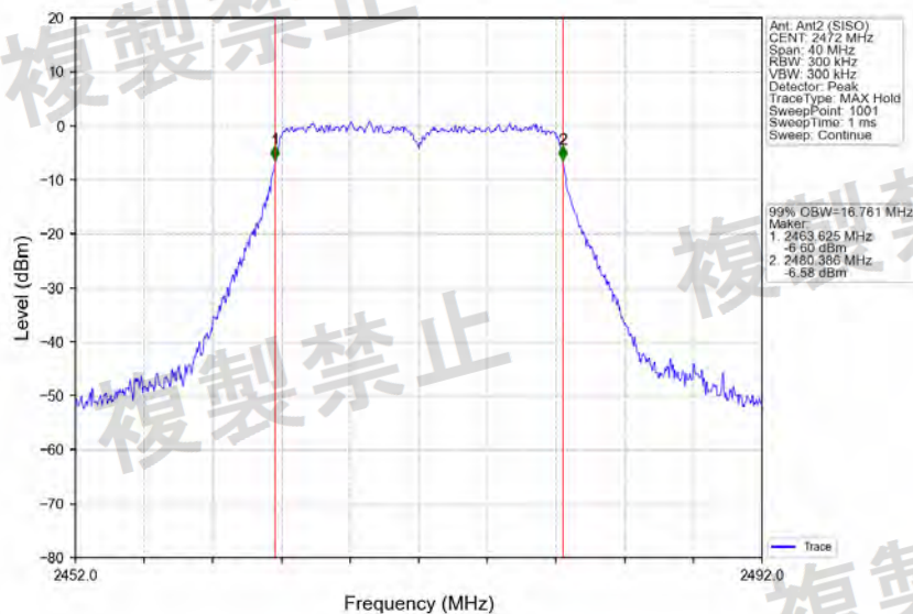
802.11g_2472MHz_Ant2 (SISO)_NTNV
