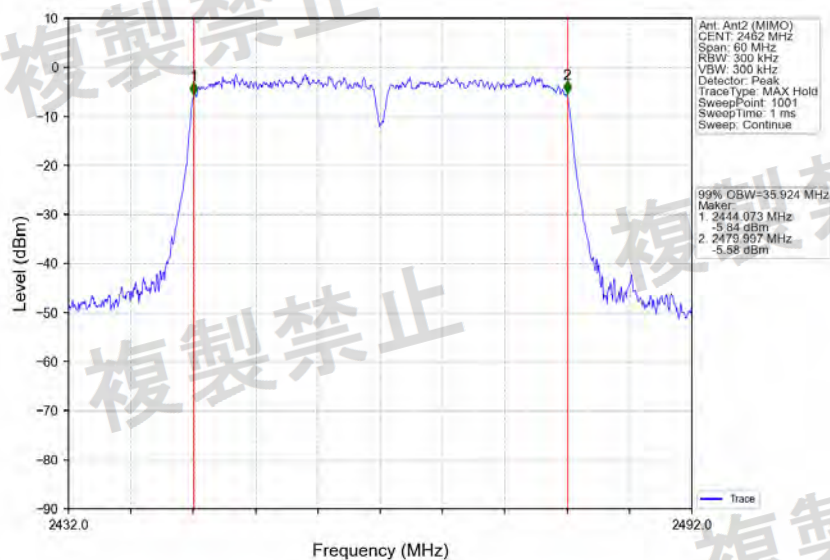
802.11n(HT40)_2462MHz_Ant2 (MIMO)_NTNV
