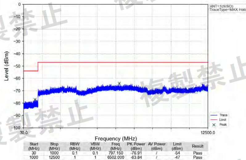
802.11g_2442MHz_Ant1 (SISO)_NTNV
