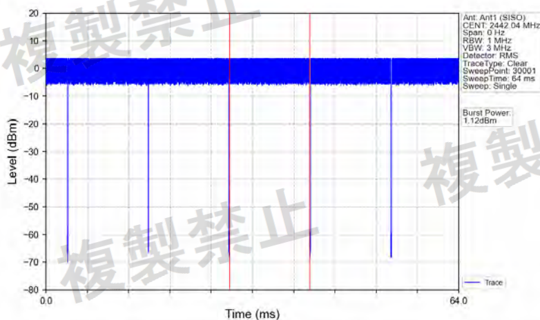
802.11b_2442MHz_Ant1 (SISO)_NTNV
