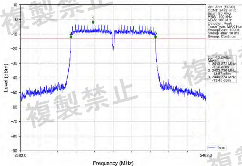
802.11n(HT40)_2422MHz_Ant1 (SISO)_NTNV
