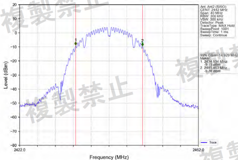
802.11b_2442MHz_Ant2 (SISO)_NTNV
