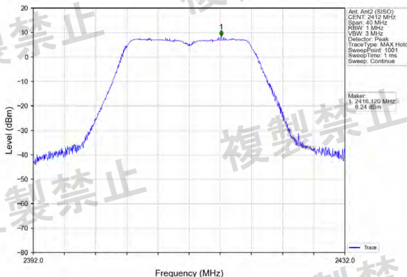
802.11g_2412MHz_Ant2 (SISO)_NTNV
