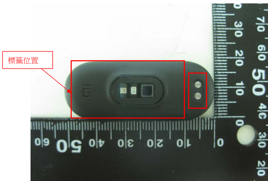
外觀照 2(充電接點)
