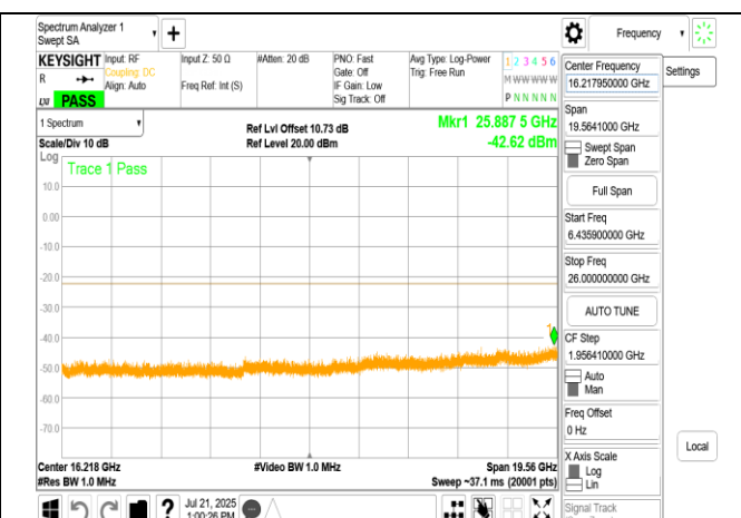
LPI 802.11ac 20MHz Chain0 6175MHz Range3
