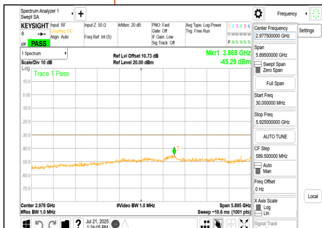
LPI 802.11ax 20MHz Chain1 5955MHz Range1
