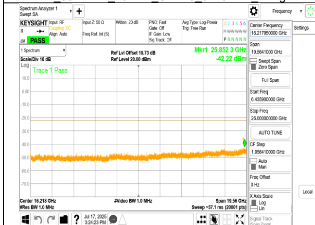
LPI 802.11be 20MHz Chain0 6415MHz Range3
