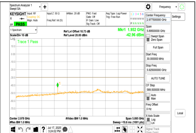
LPI 802.11be 20MHz Chain0 6415MHz Range1
