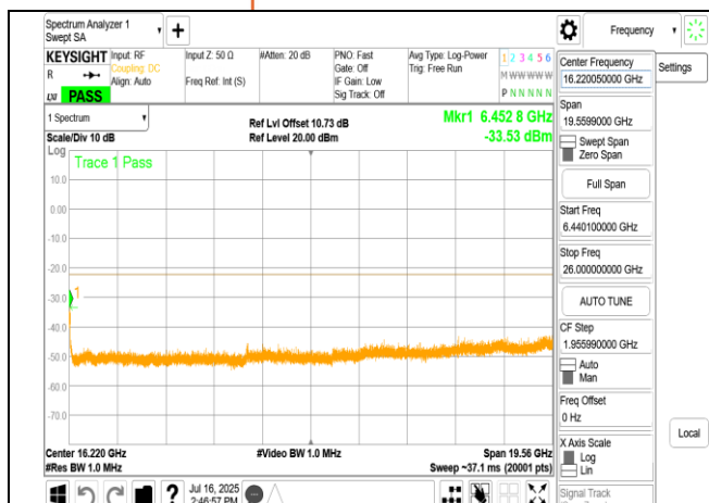
LPI 802.11ac 40MHz Chain1 6405MHz Range3
