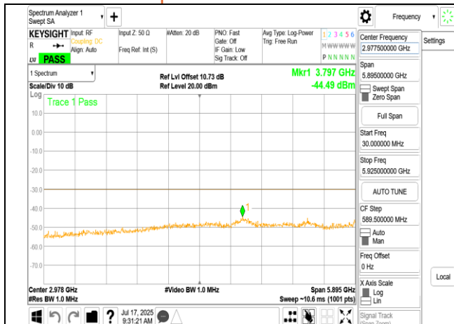
LPI 802.11ac 160MHz Chain0 6185MHz Range1
