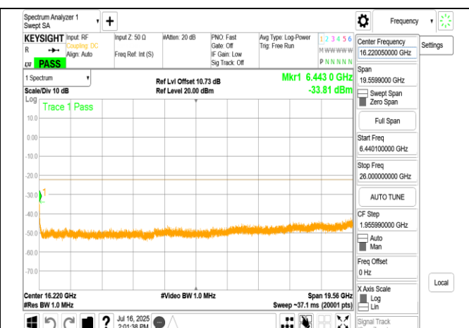
LPI 802.11n 40MHz Chain1 6405MHz Range3
