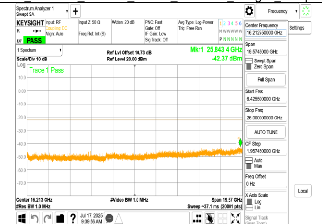
LPI 802.11ac 160MHz Chain1 6025MHz Range3
