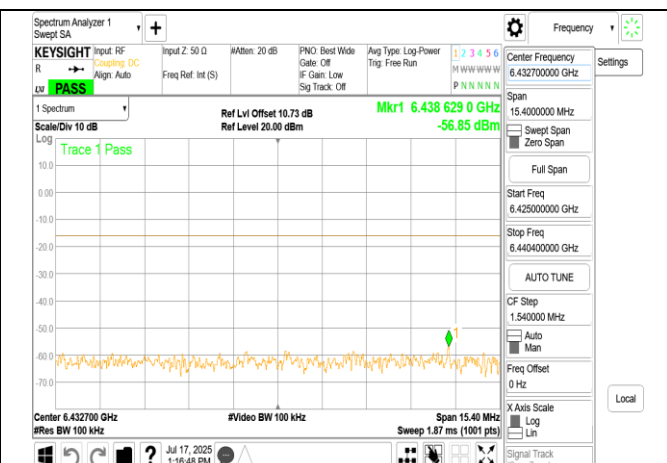
LPI 802.11ax 40MHz Chain1 6165MHz Range2
