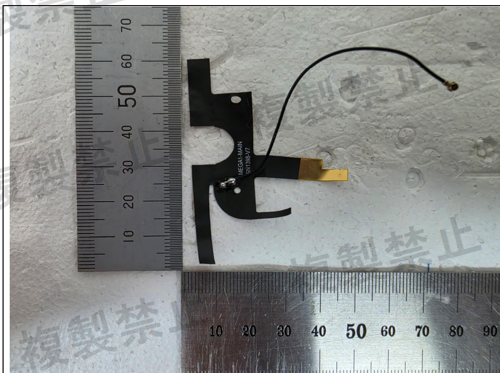
< LTE Antenna >
