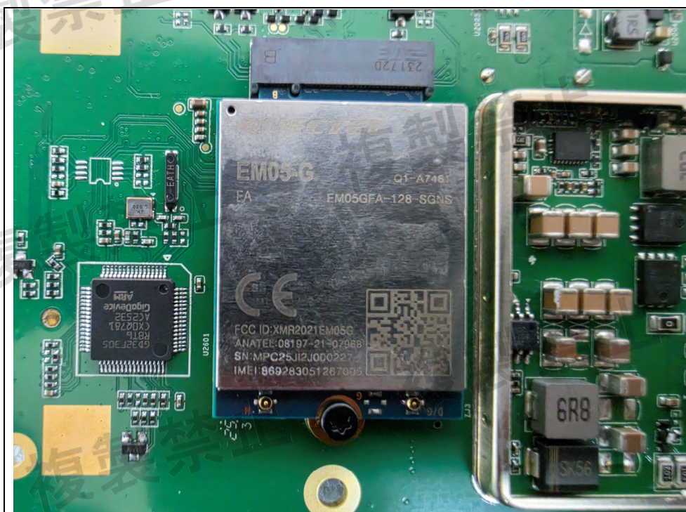
< LTE module >
