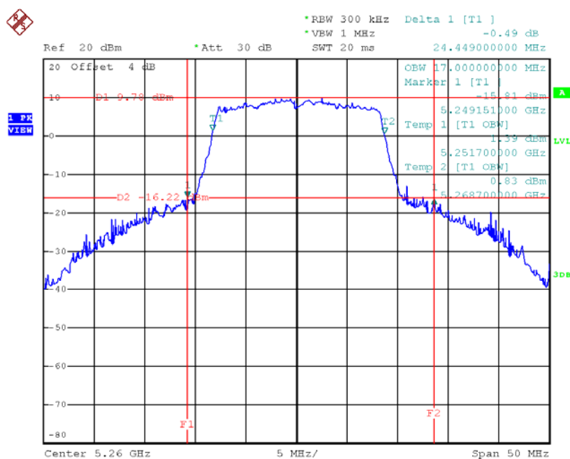
IEEE 802.11a / 5260 MHz
