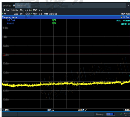
NTVN-11AC40SISO-Ant1-5670-30~5460-PASS
