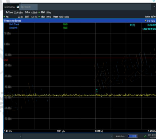
NTVN-11AC40SISO-Ant1-5670-5460~5470-PAS
