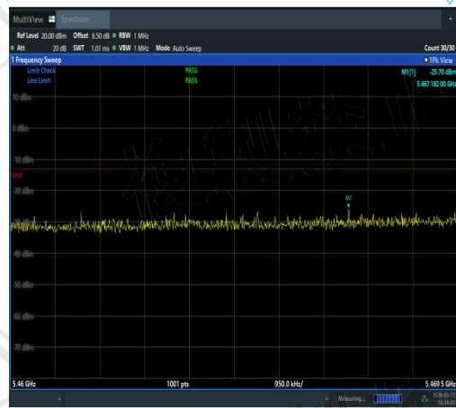
NTVN-11AC80SISO-Ant1-5530-5460~5469.5-PA SS
