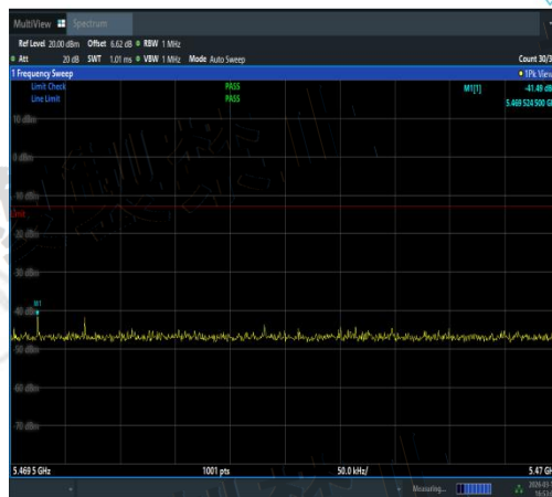
NTNV-11AC80SISO-Ant2-5690-5469.5~5470-PA SS
