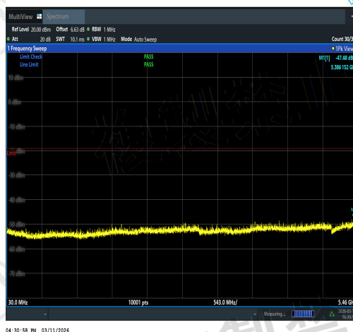
NTVN-11AC40SISO-Ant3-5710-30~5460-PASS
