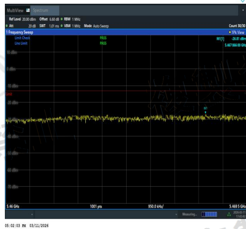
NTVN-11AC80SISO-Ant1-5530-5460~5469.5-PA SS
