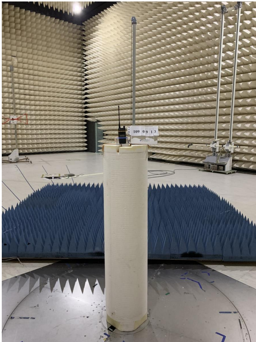
1GHz 以上輻射電場強度最大干擾擺置實際照片(正面)
