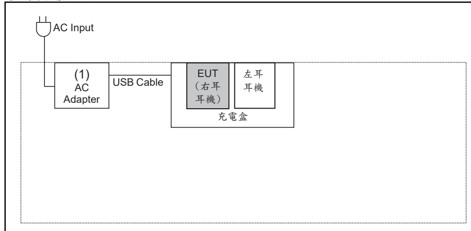
電源傳導干擾測試配置
