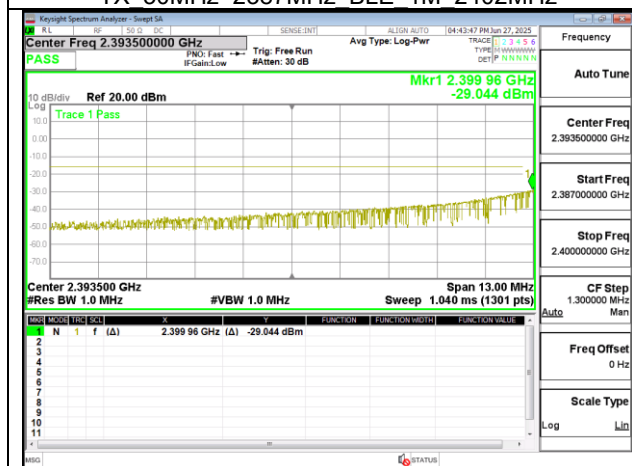
TX 2387MHz~2400MHz BLE 1M 2402MHz
