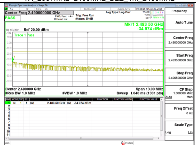
TX 2483.5MHz~2496.5MHz BLE 1M 2480MHz.png
