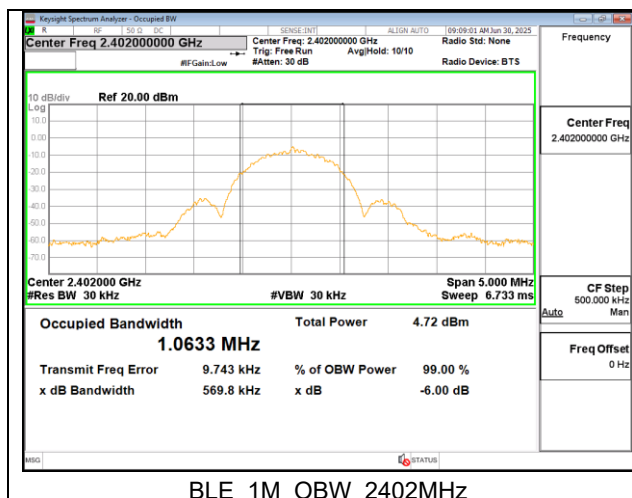
BLE 1M OBW 2402MHz
