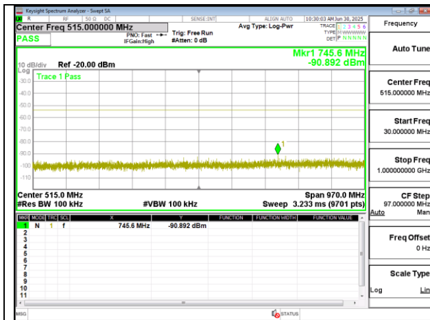
RX Below 1GHz BLE 1M 2402MHz
