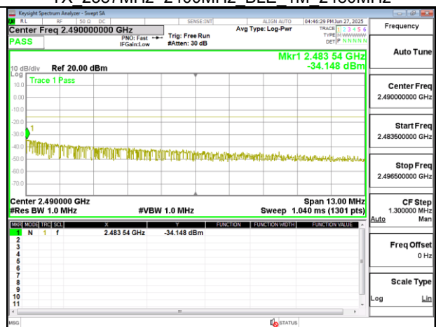
TX 2483.5MHz~2496.5MHz BLE 1M 2480MHz
