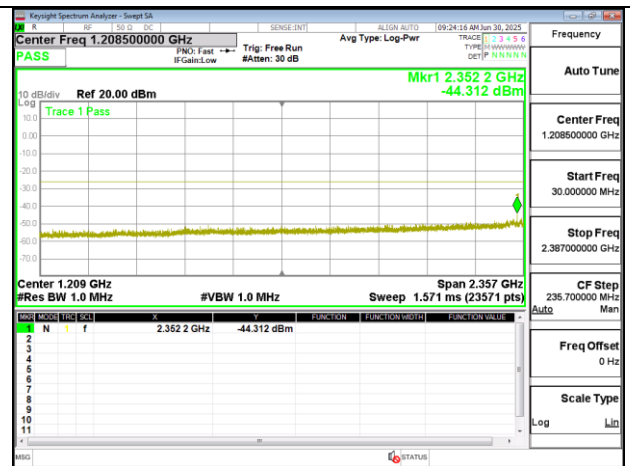
TX 30MHz~2387MHz BLE 1M 2480MHz
