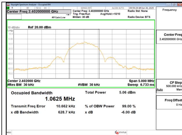
BLE 1M OBW 2402MHz
