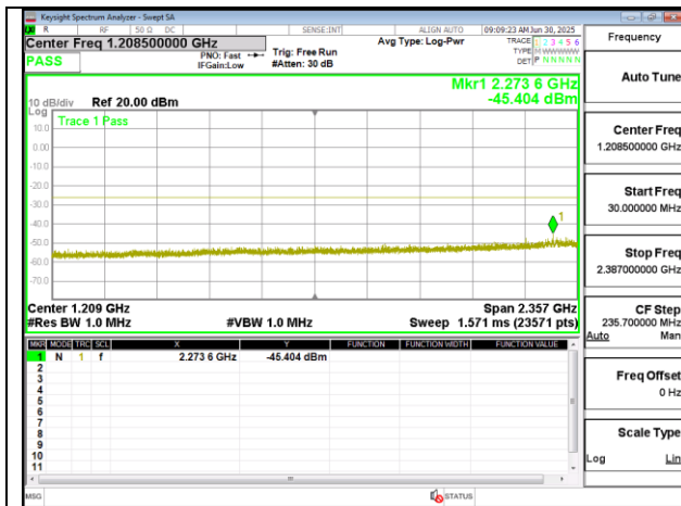
TX 30MHz~2387MHz BLE 1M 2402MHz
