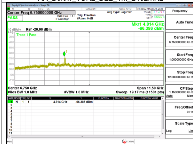
RX Above 1GHz BLE 1M 2402MHz
