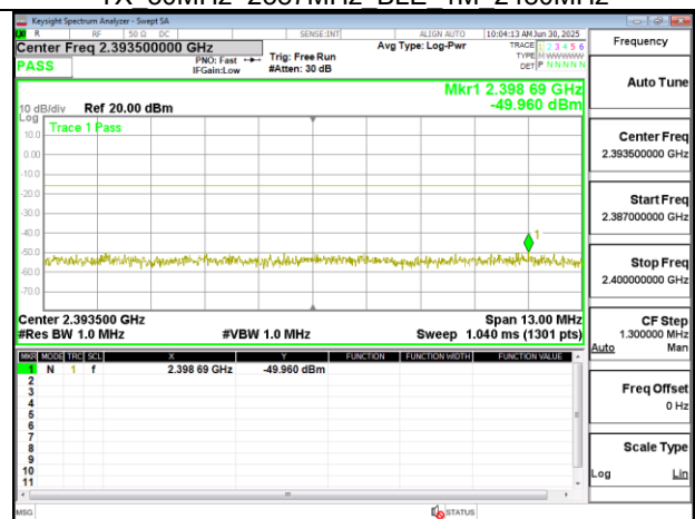
TX 2387MHz~2400MHz BLE 1M 2480MHz
