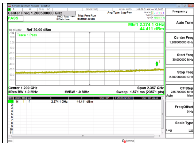
TX 30MHz~2387MHz BLE 1M 2402MHz
