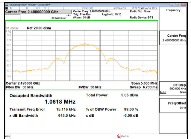
BLE 1M OBW 2480MHz
