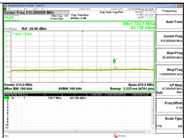
RX Below 1GHz BLE 1M 2480MHz
