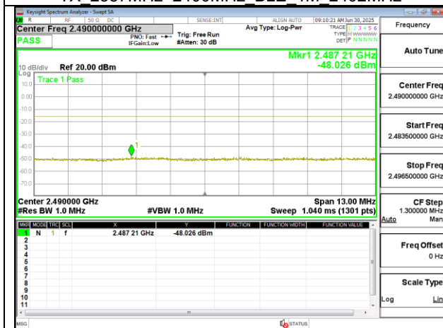
TX 2483.5MHz~2496.5MHz BLE 1M 2402MHz
