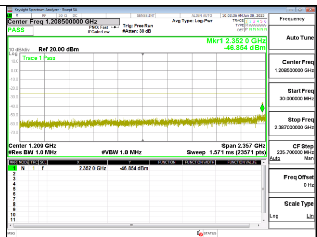
TX 30MHz~2387MHz BLE 1M 2480MHz
