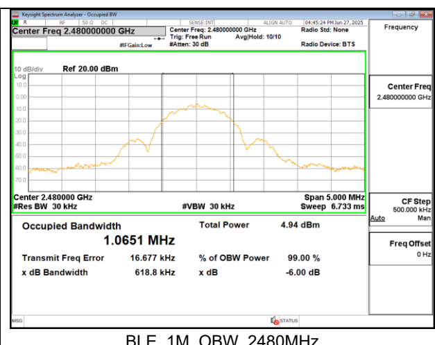
BLE 1M OBW 2480MHz
