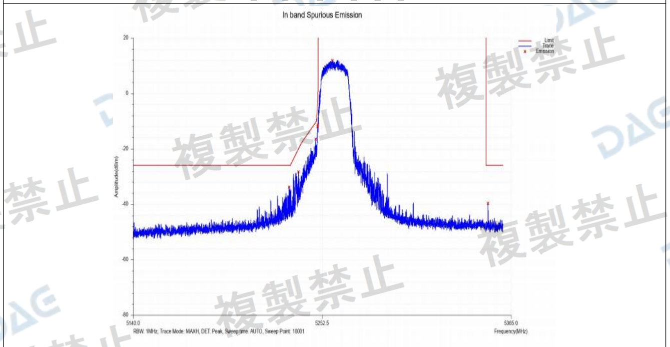
In_band_NVNT_ANT1_802_11a_5260
