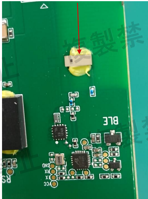
BLE ANT
