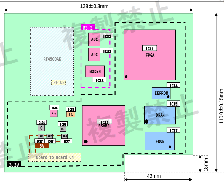
RF-PKG部品配置図 (1 / 2)
