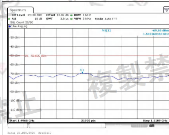
1496.6-1510.9_new
