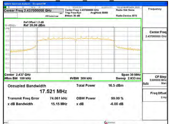
發射頻寬 6dB 之要求
