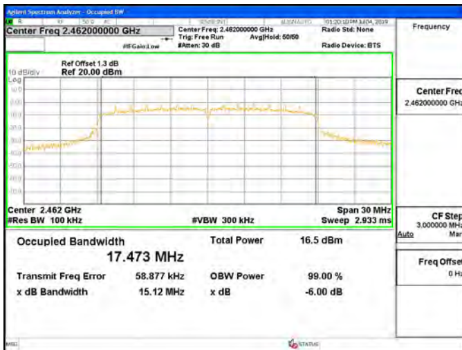
發射頻寬 6dB 之要求
