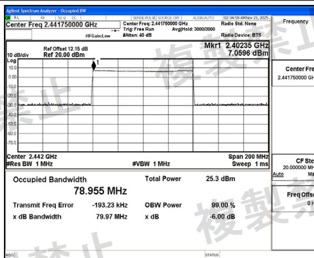
NTNV_2DH5_Ant1_Hop
