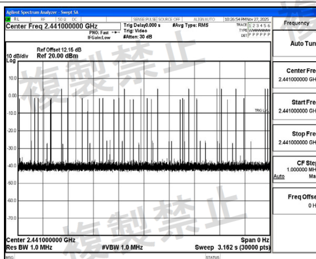
NTNV_3DH1_Ant1_Hop
