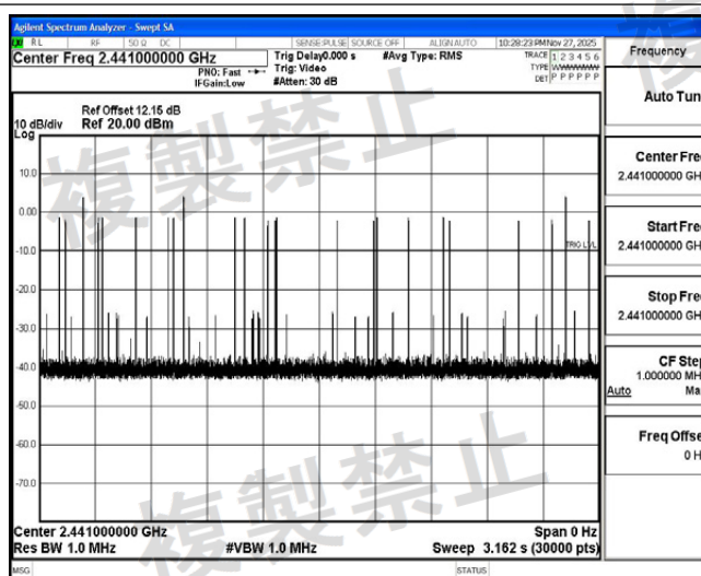
NTLV_3DH1_Ant1_Hop
