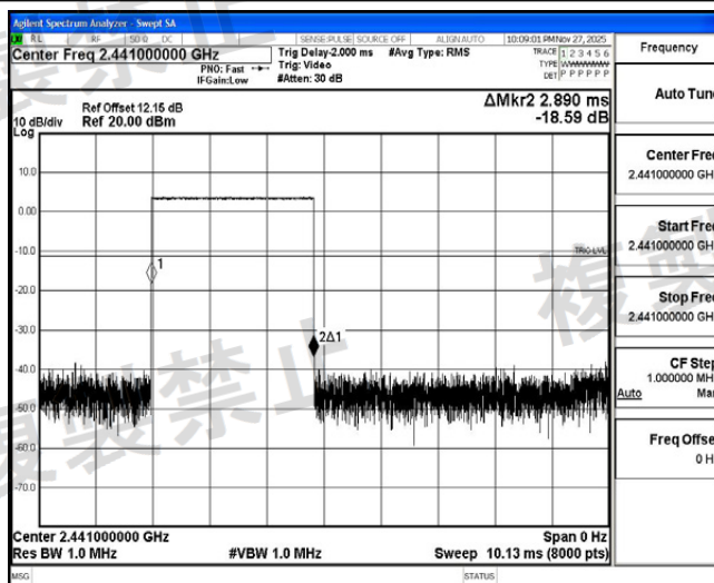
NTNV_DH5_Ant1_Hop
