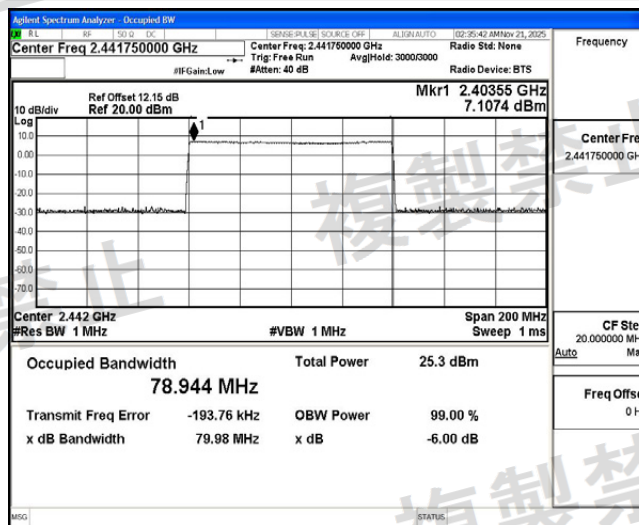
NTHV_2DH5_Ant1_Hop
