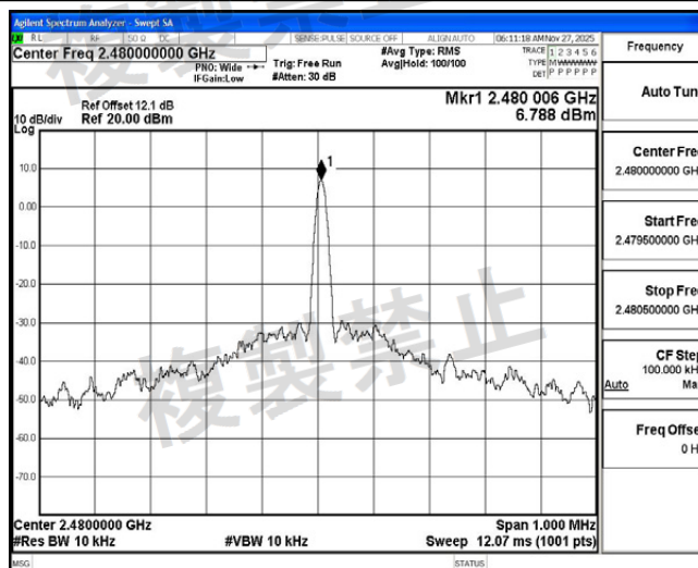
NTNV_DH5_Ant1_2480
