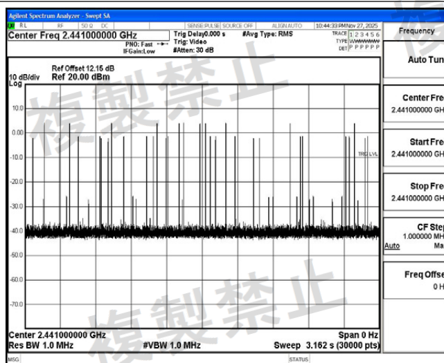
NTLV_DH1_Ant1_Hop
