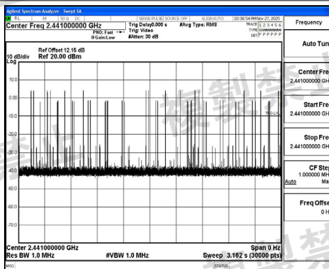
NTLV_2DH5_Ant1_Hop
