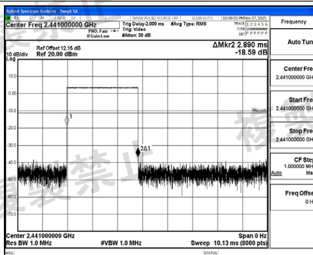
NTLV_3DH5_Ant1_Hop
