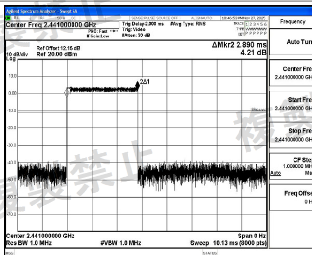
NTHV_3DH5_Ant1_Hop
