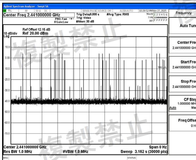
NTHV_3DH1_Ant1_Hop
