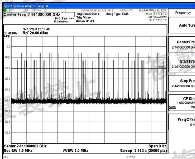
NTNV_DH3_Ant1_Hop
