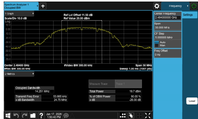
90% OBW
