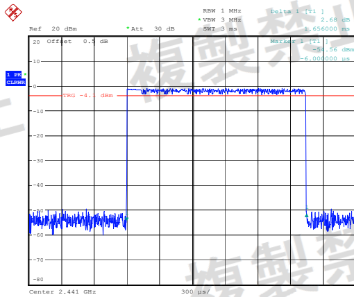
\pi/4 -DQPSK_Hopping_2DH3
