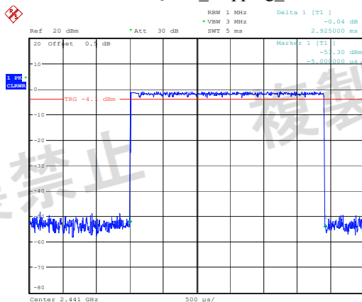
\pi/4 -DQPSK_Hopping_2DH5
