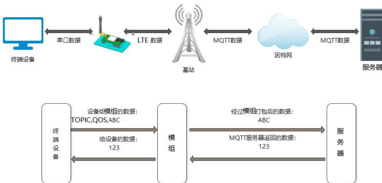
图 6 MQTT 模式通信示意图
