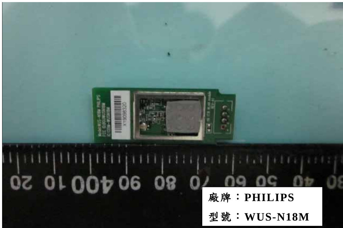
RF模組外觀照
