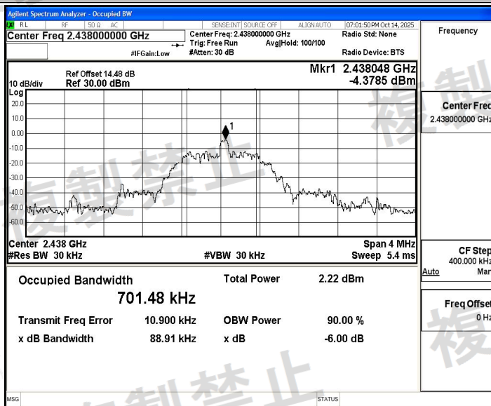
NTNV_2.4G_Ant1_2438
