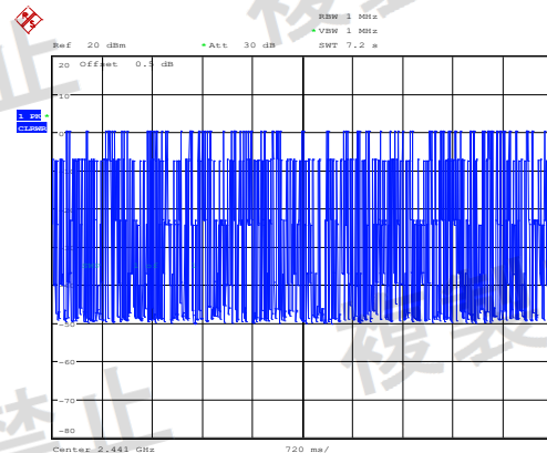
GFSK_Hopping_AFH_DH5
