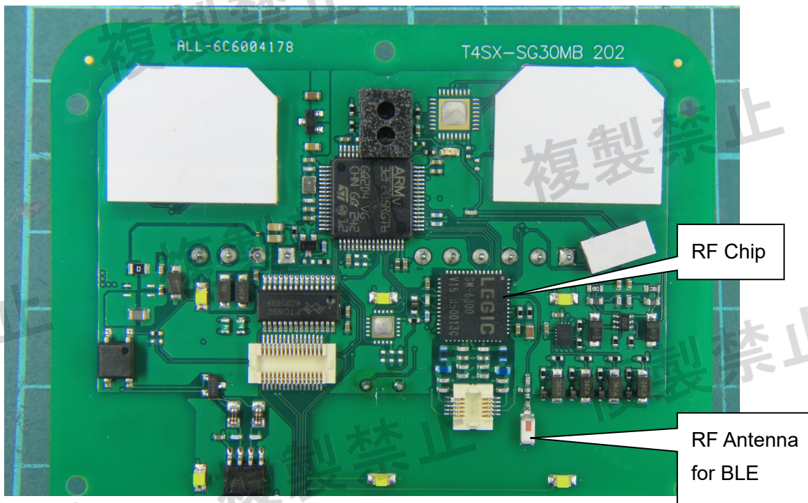
(16) EUT Photo
