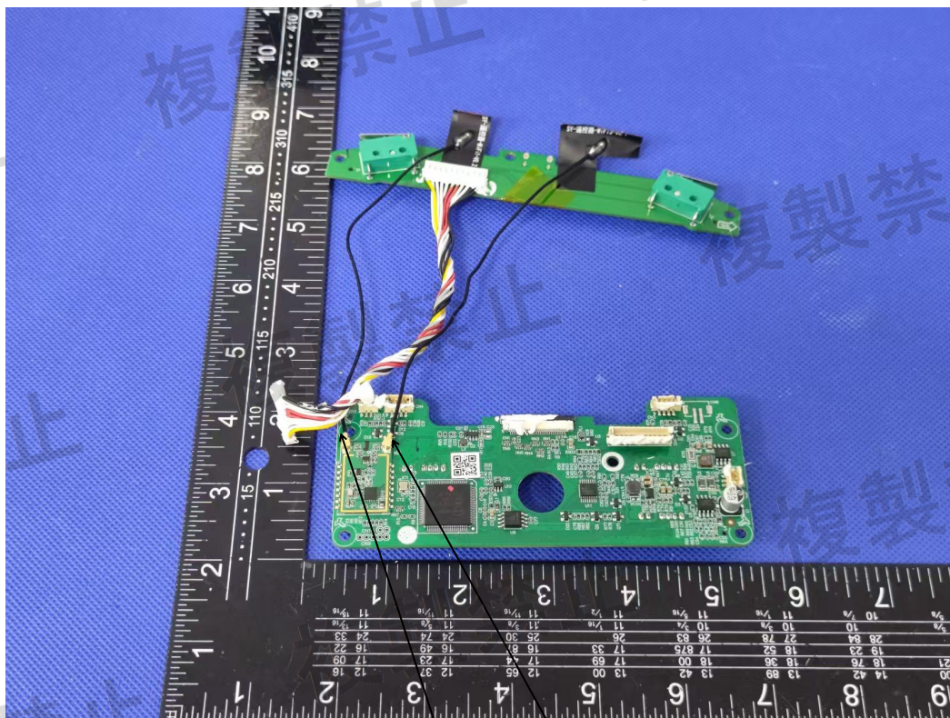
ANT1 ANT2
