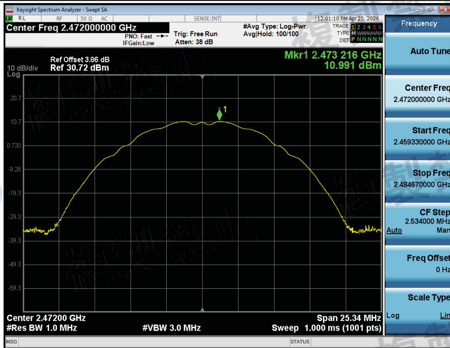
2_Antena_Power_NVNT_ANT1_802_11b_2472
