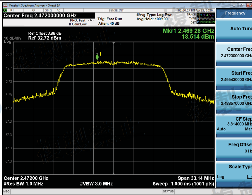
2_Antena_Power_NVNT_ANT1_802_11g_2472
