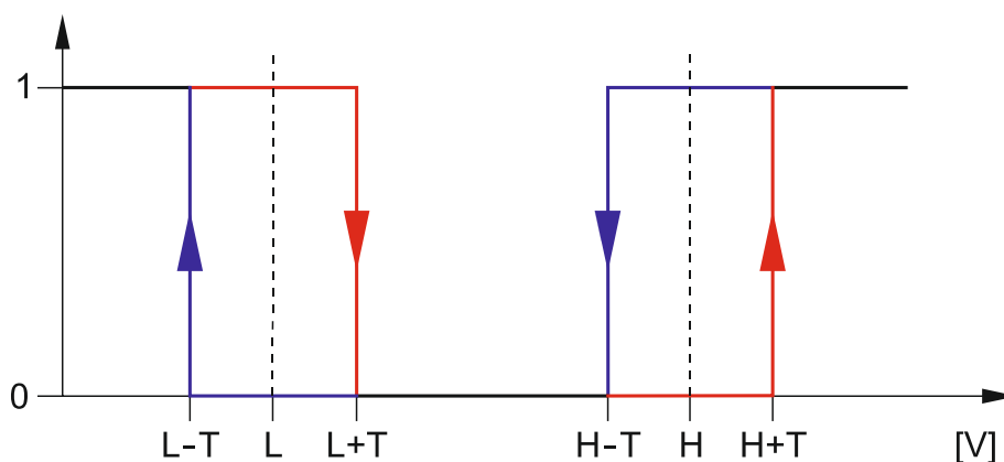
Obr. 21. Význam funkce analogového vstupu. 0 – normální stav (bez narušení), 1 – dosažena úroveň (narušení), L-T – spodní úroveň mínus tolerance, L – spodní úroveň, L+T – spodní úroveň plus tolerance, H-T – horní úroveň mínus tolerance, H – horní úroveň, H+T – horní úroveň plus tolerance.
