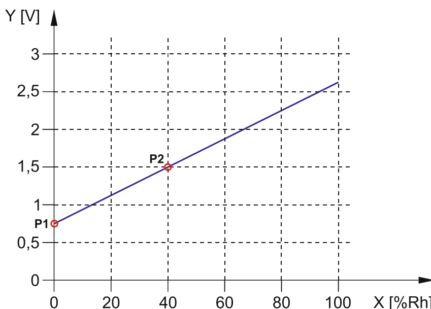
Obr. 22. Příklad lineární charakteristiky senzoru relativní vlhkosti vzduchu.
