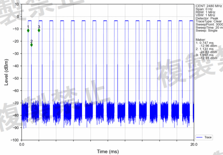
GFSK_DH1_2480MHz_Ant1_NTNV
