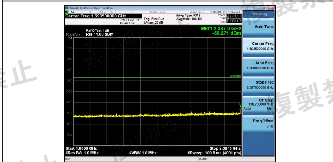
NTNV-11B-Ant1-2472-1000~2387-PASS
