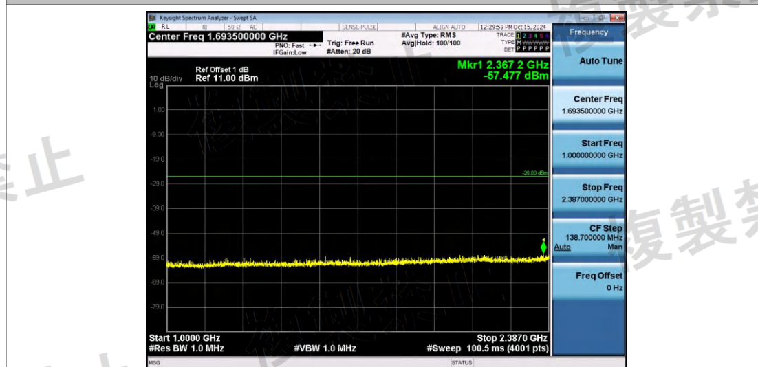
NTNV-11G-Ant1-2472-1000~2387-PASS
