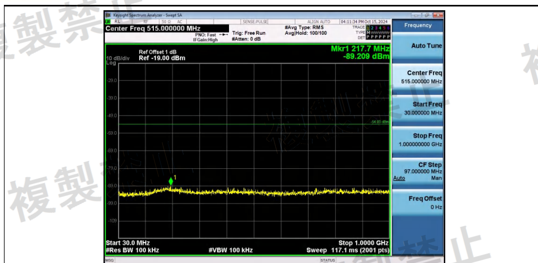
NTNV-11G-Ant1-2412-30~1000-PASS
