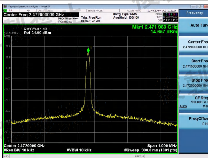
NTVN-CW-Ant1-2472-PASS
