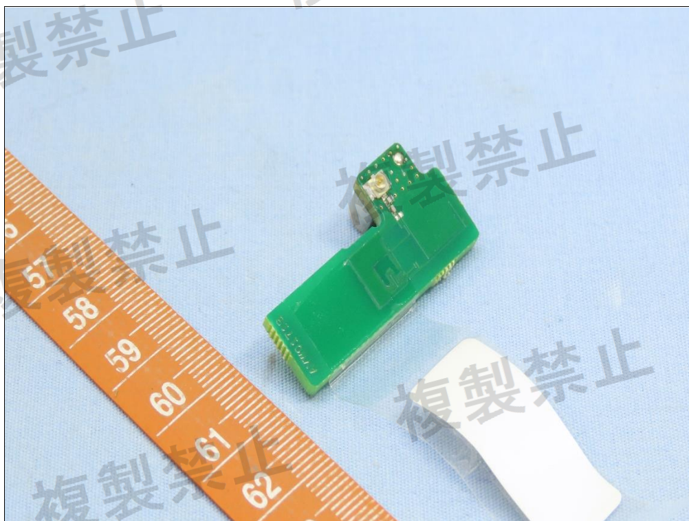
Antenna 10 (Brand: HAIVISION / Model: XANTIGUA_WIFI_AUX)
