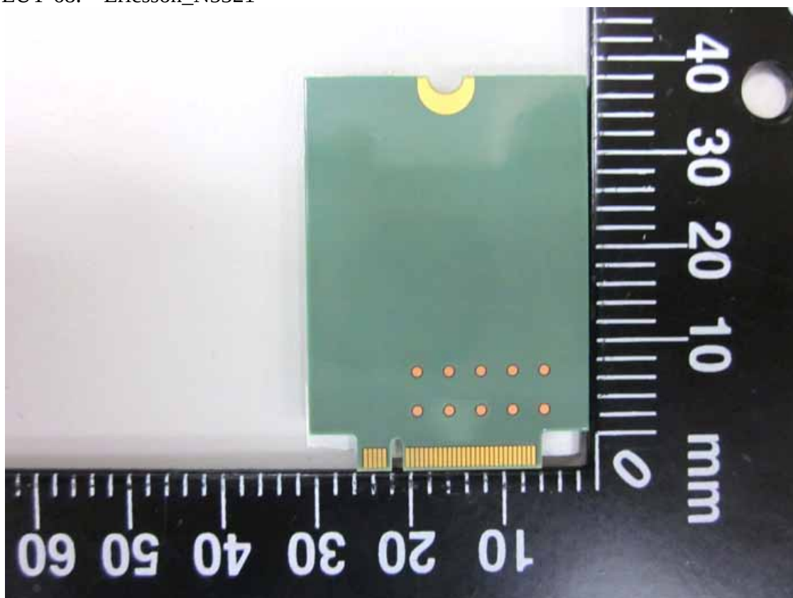
EUT-68. Ericsson_N5321
