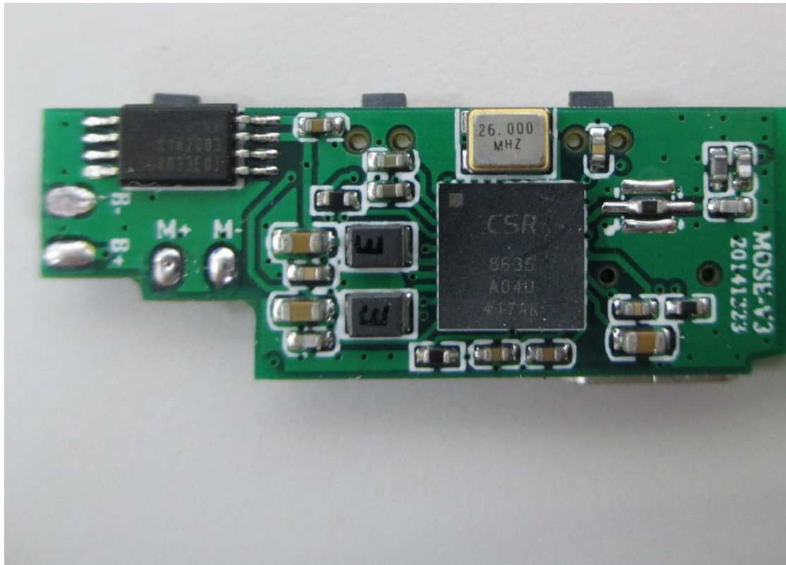
CSR CSR8635 正面照
