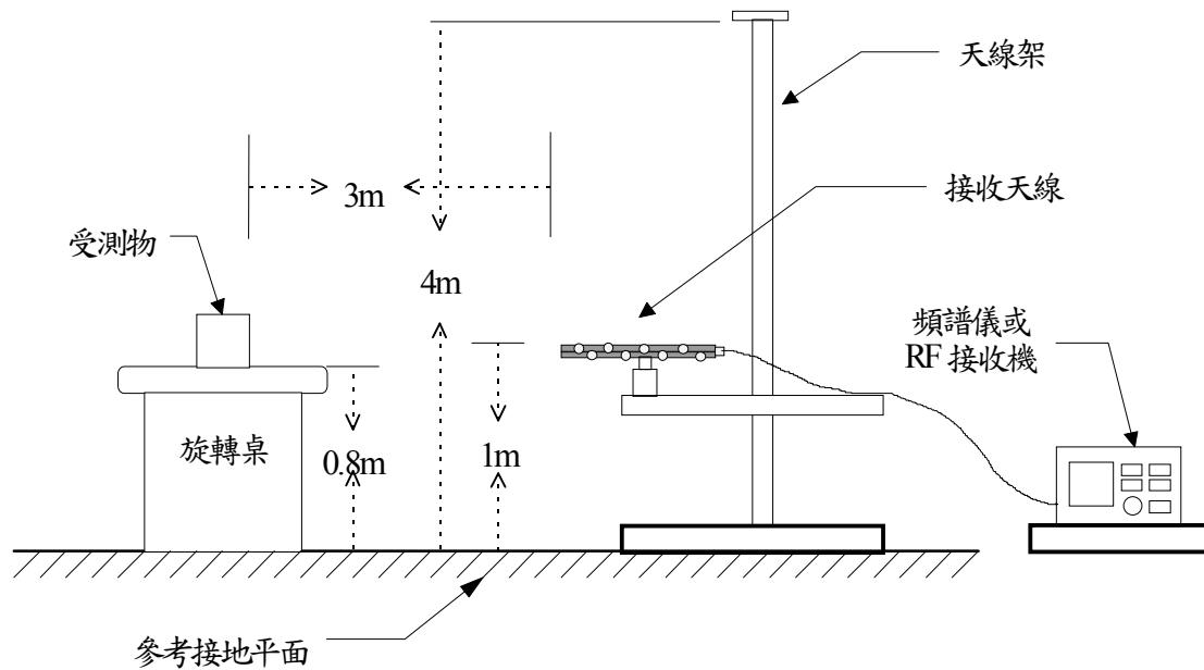
圖 2: 量測頻率低於1GHz之測試配置 (RE01)
