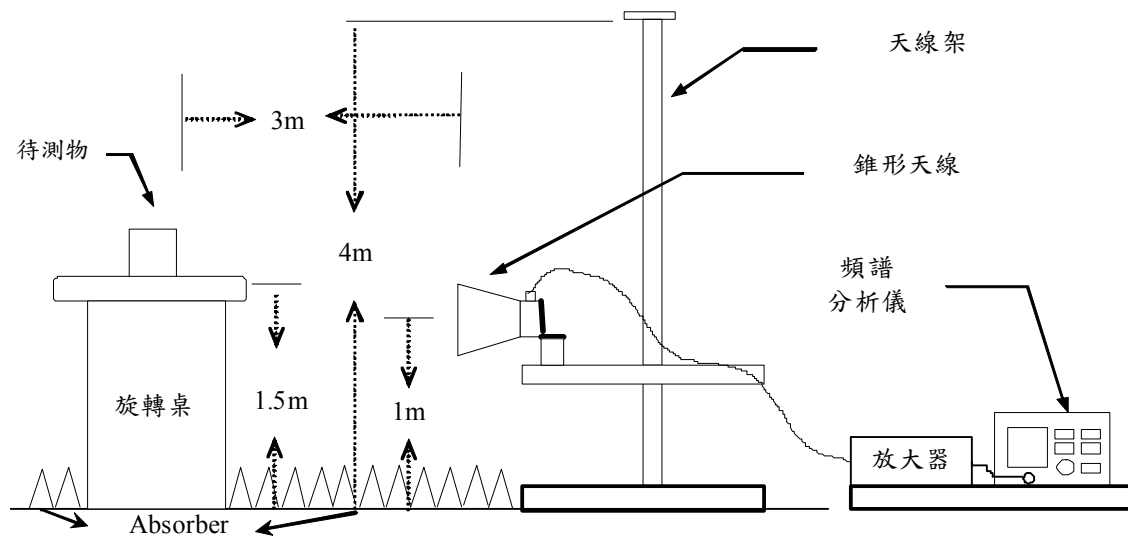
圖 3: 量測頻率高於1GHz之測試配置 (RE01)
