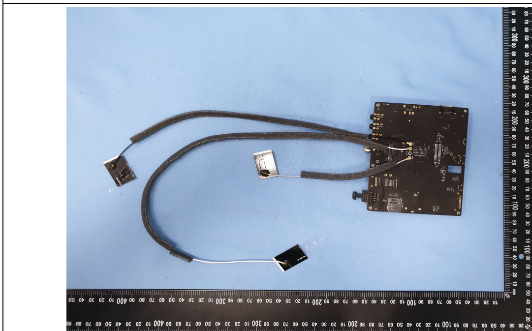
治具照
