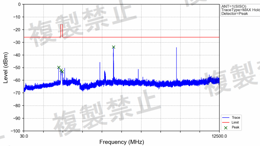
GFSK DH5 2441MHz Ant1 NTLV
