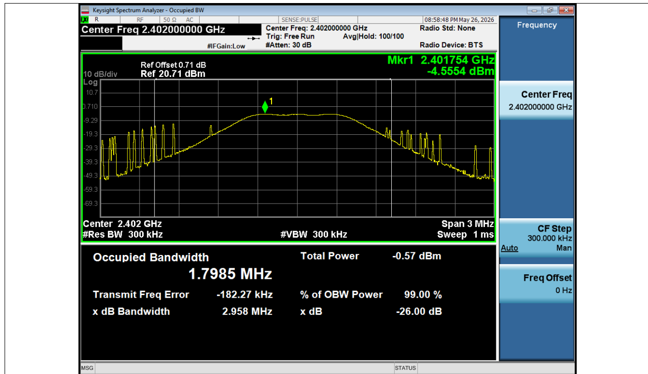
OBW NVNT BLE 1M 2402MHz Ant1
