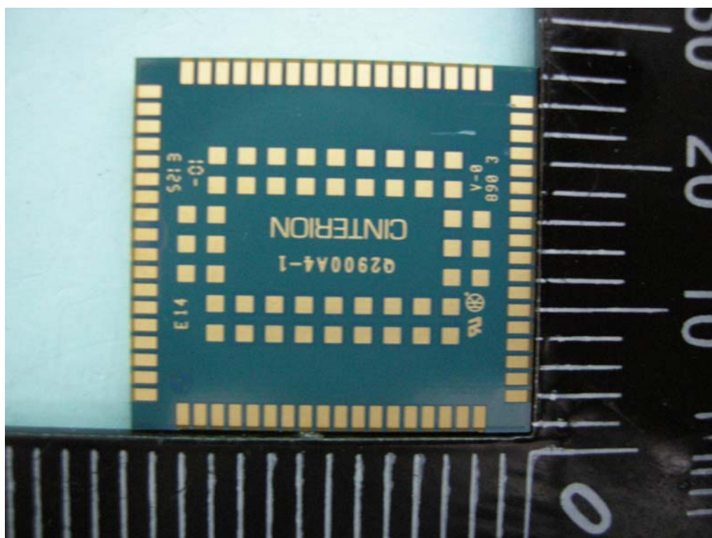
廠牌：CINTERION 型號：EHS6 照片二：背面照
