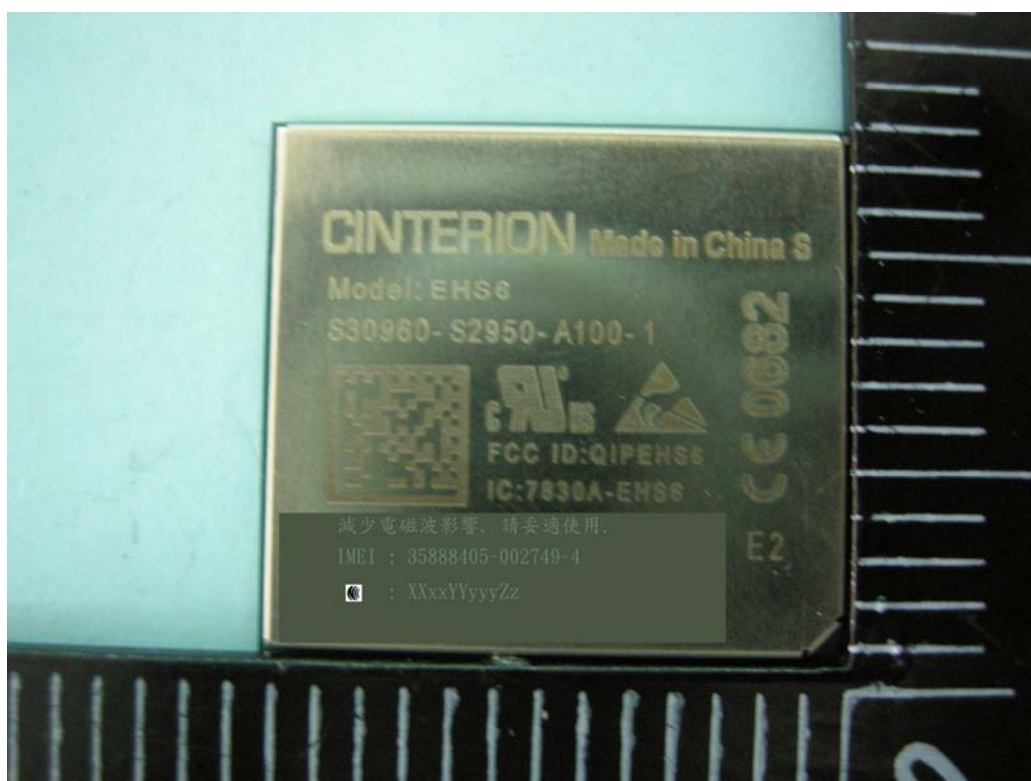
廠牌：CINTERION 型號：EHS6 照片一：正面照
