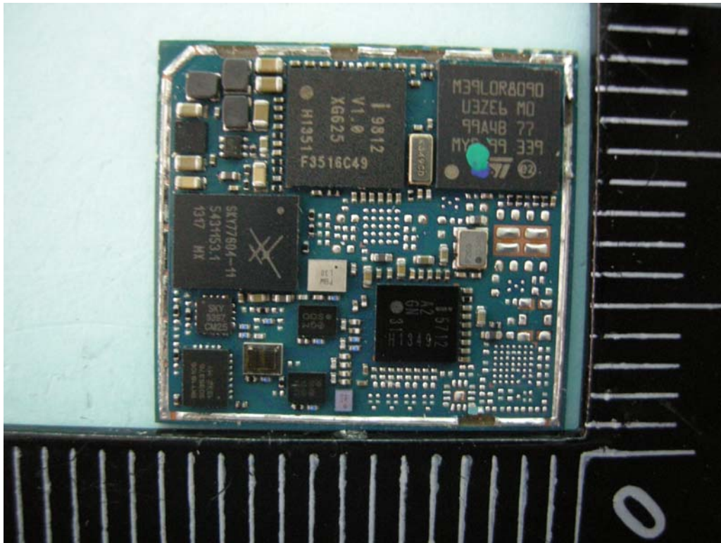
廠牌：CINTERION 型號：EHS6 照片三：內部照
