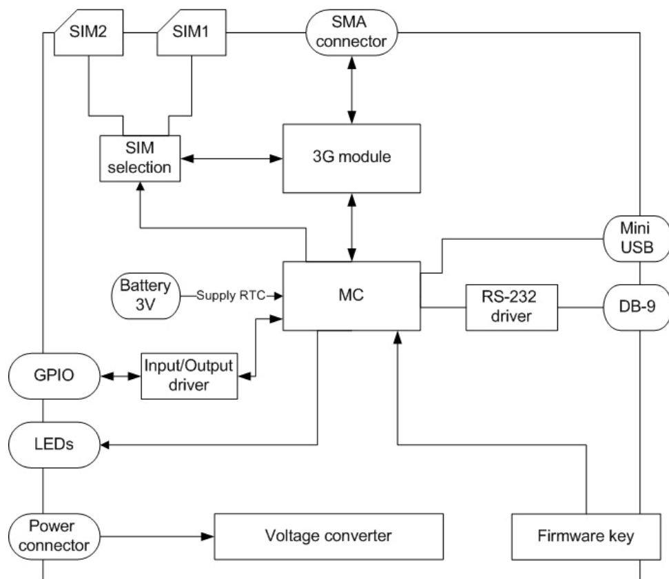
Рис. 2.1 Функциональная схема ATM
