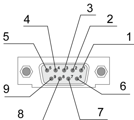
Рис. 2.5 Разъем DB9
