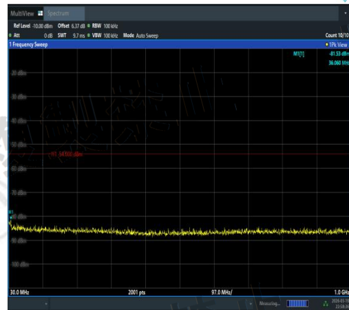
NTVN-11AC80SISO-Ant2-5210-30~1000-PASS
