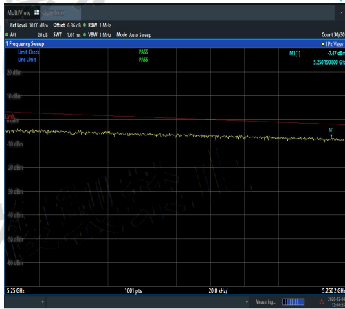
NTVN-11AX20MIMO-Ant1-5240-5250~5250.2-P ASS
