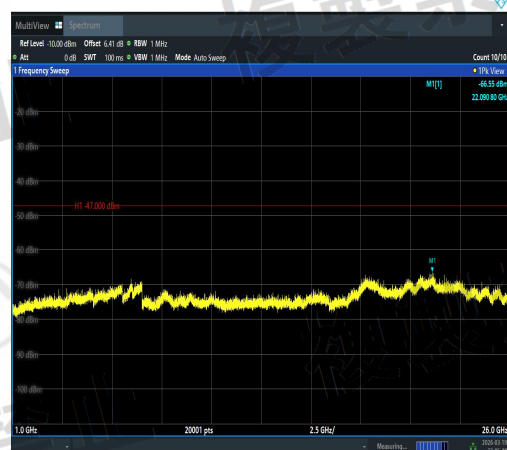
NTVN-11AC80SISO-Ant3-5210-1000~26000-PA SS
