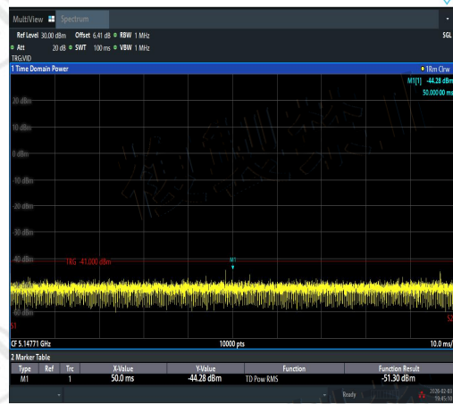
NTNV-11AC80SISO-Ant3-5210-5132.5~5150-PA
