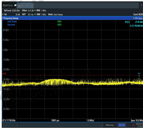
NTNV-11AC80SISO-Ant2-5210-30~5123.2-PAS
