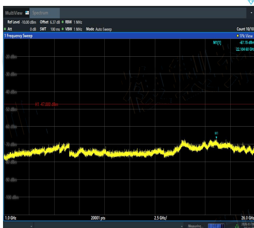
NTVN-11AC80SISO-Ant2-5210-1000~26000-PA SS
