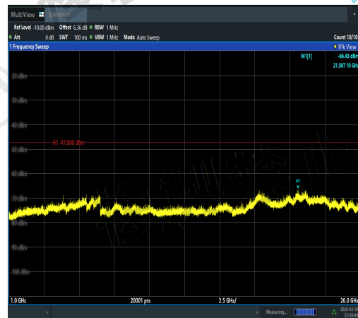
NTVN-11AC80SISO-Ant1-5210-1000~26000-PA SS
