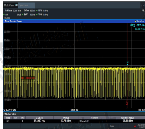
NTVN-11AX20MIMO-Ant1-5240-5250~5250.2-P ASS
