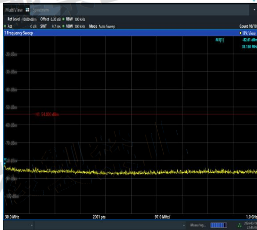
NTVN-11A-Ant1-5220-30~1000-PASS
