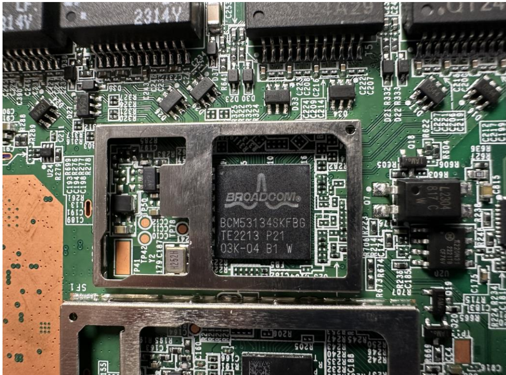
(21) EUT Photo
