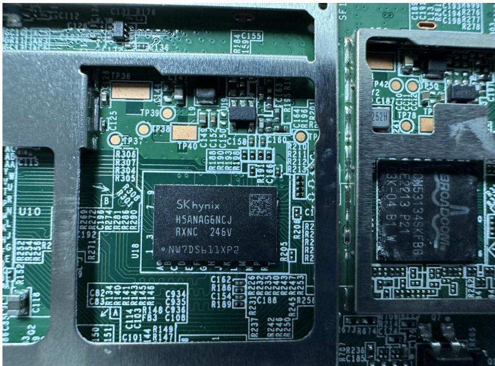
(20) EUT Photo
