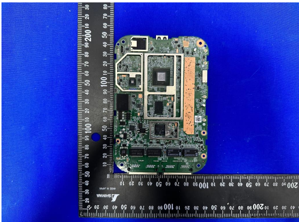
(18) EUT Photo
