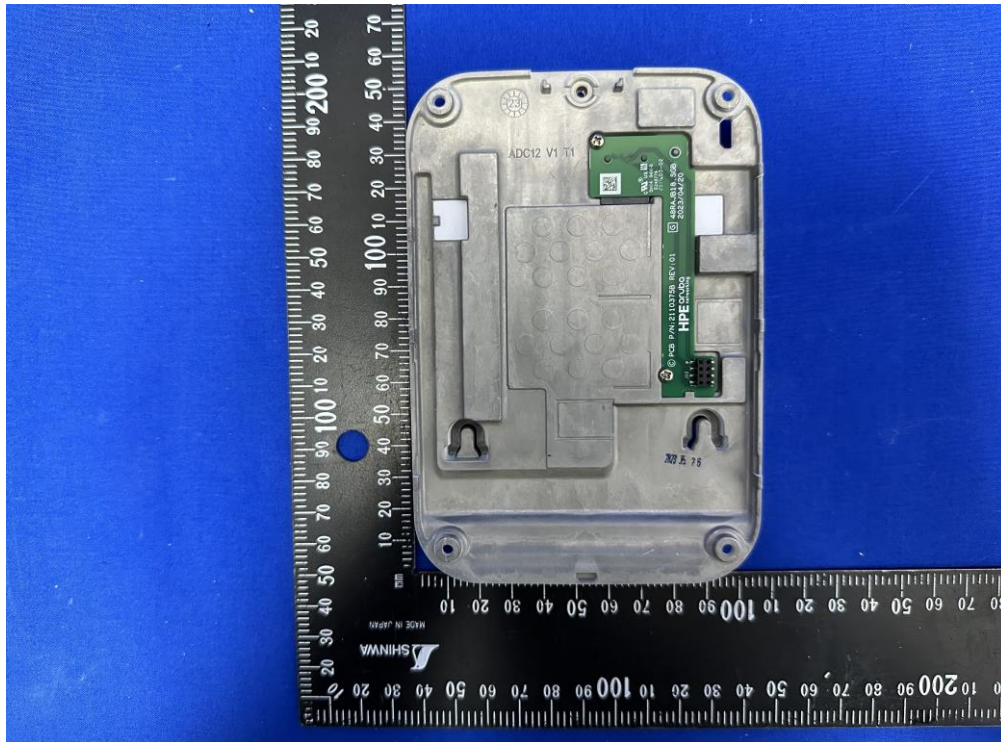
EUT Photo
