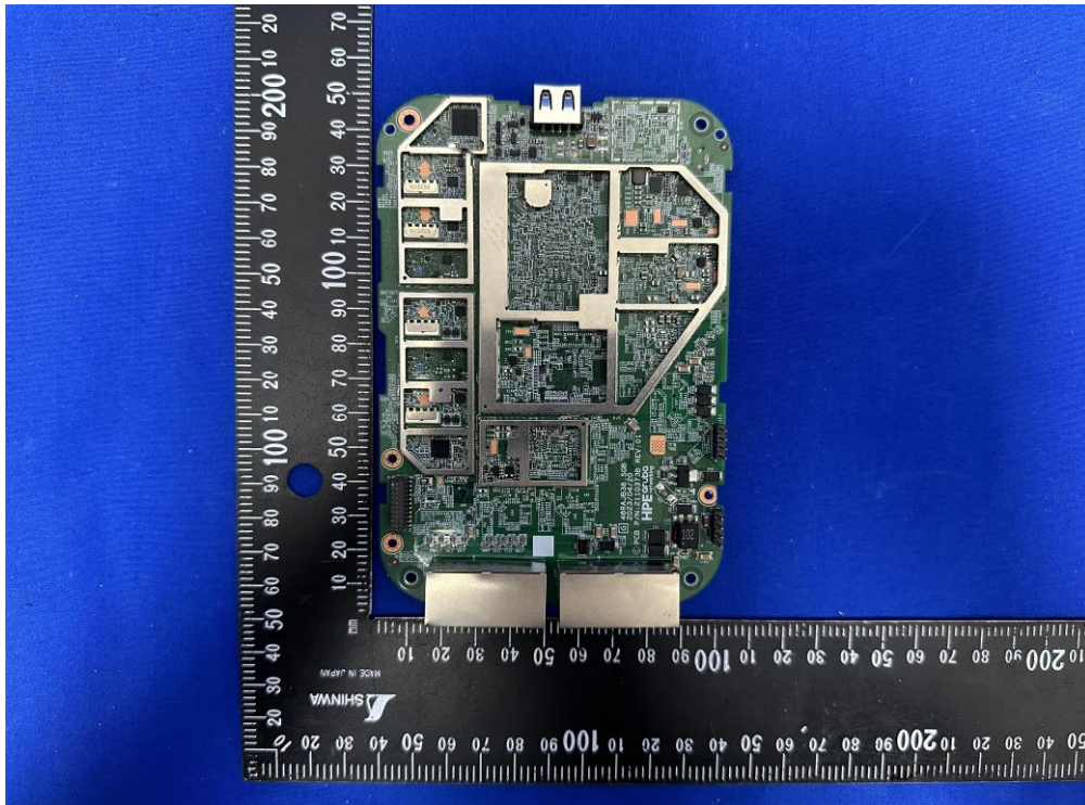
(16) EUT Photo
