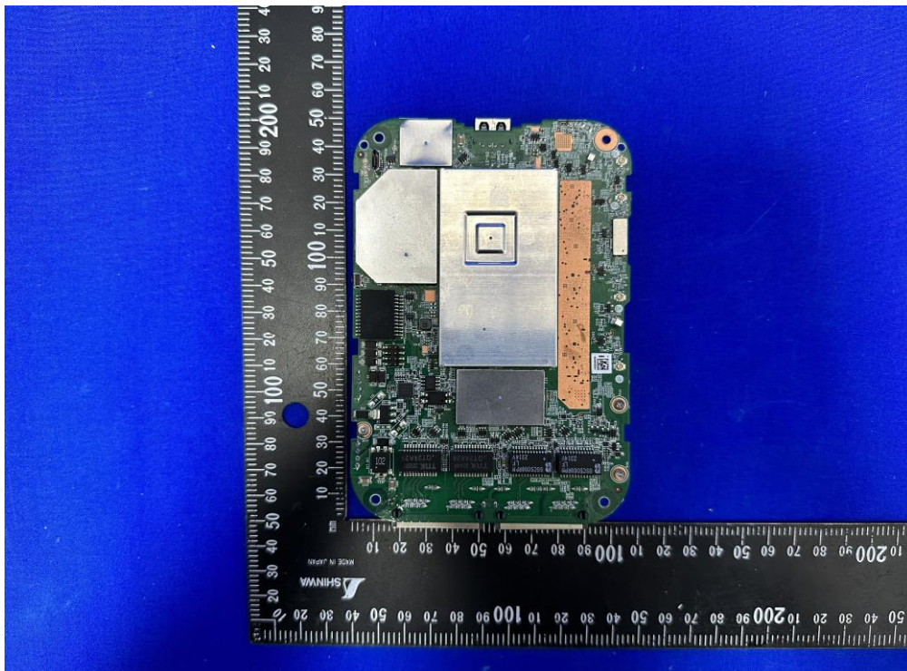
(5) EUT Photo
