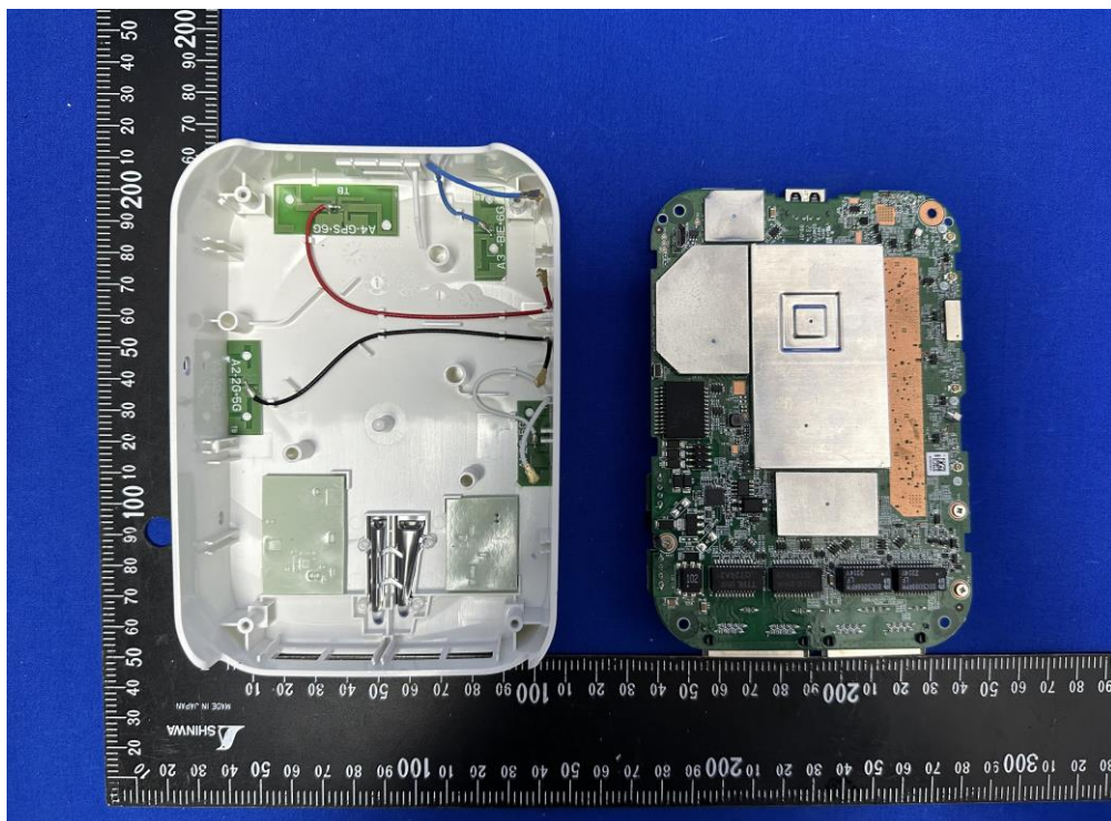
(3) EUT Photo
