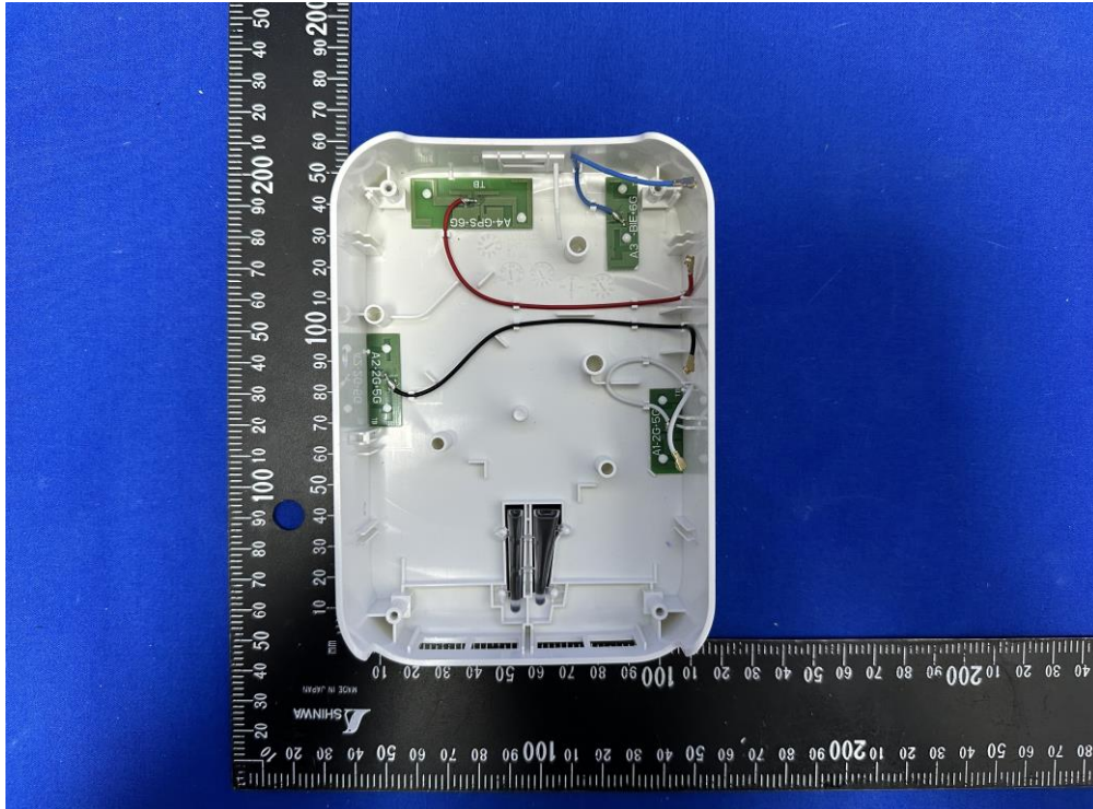
(4) EUT Photo
