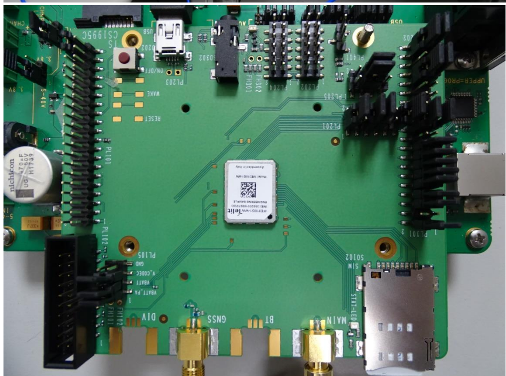
EUT 近照
